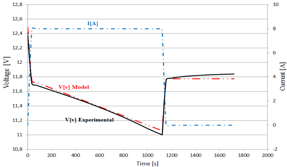
Figure III-26: Modèle de performance comparé au modèle issu de la caractérisation expérimentale. Les deux signaux sont assez proches du fait d'une très bonne estimation des paramètres du modèle.
