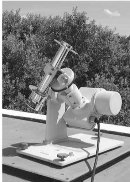
(c) Pyrhéliomètre Eppley
