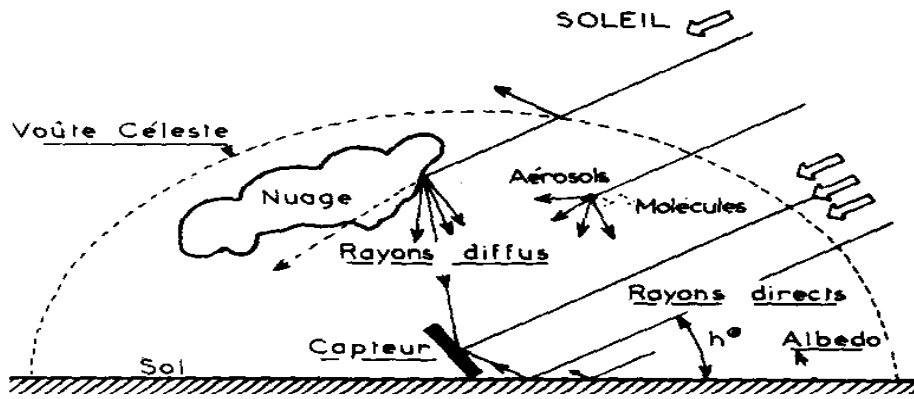
Figure II-8: Rayonnement solaire[37]
