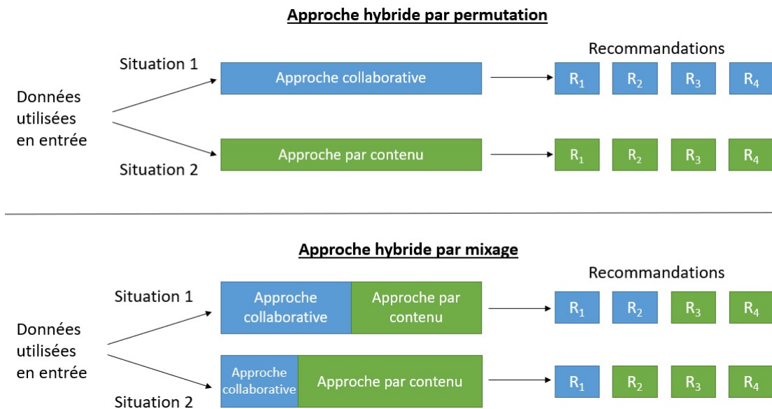
FIGURE 1.2 – Exemple de modèles de recommandation hybrides [?]
