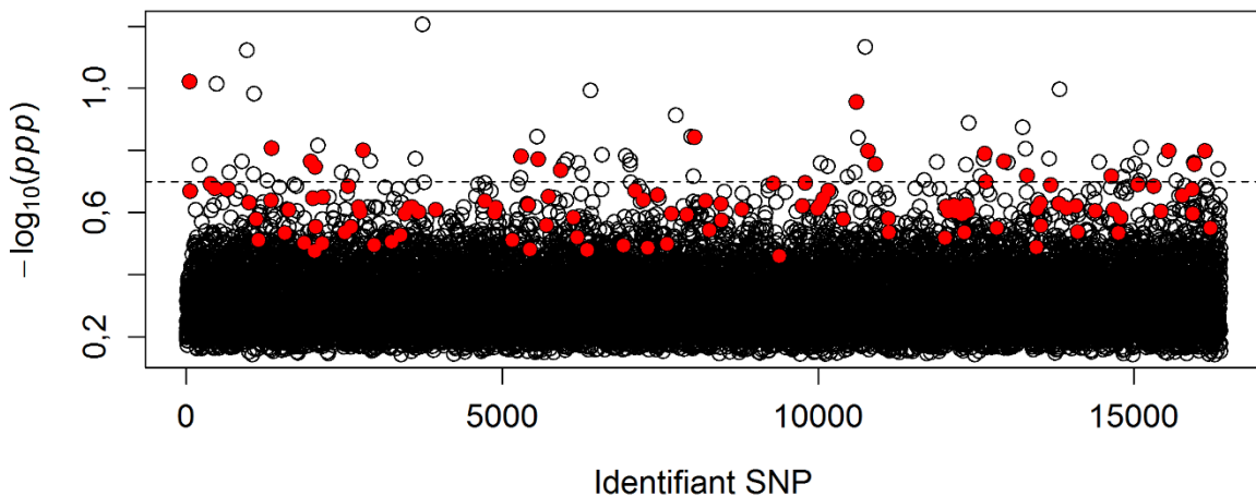
Figure VI-10. Soixante-seize SNP candidats à la sélection ont été identifiés au moyen de KimTree au sein des lignées expérimentales du dispositif EFFICACE. Les p-values postérieures prédictives ( PPP-values ), qui permettent de quantifier la probabilité d'un rôle de la sélection au sein de populations apparentées (Gautier et al. , 2010), ont été calculées au moyen de KimTree (Gautier & Vitalis, 2013). (a) Diagramme de Tukey des 16370 PPP-values associées au jeu de marqueurs obtenu par génotypage des lignées expérimentales du dispositif EFFICACE. Le point rouge indique la moyenne des PPP-values . (b) Le graphique indique en ordonnée -\log_{10}(ppp) où ppp désigne la PPP-value . Pour être candidat, un SNP doit être associé à ppp \leq 0,2 (tirets, -\log_{10}(ppp) \approx 0,7 ), un seuil de significativité qui semble constituer un bon compromis entre puissance et contrôle du taux de faux-positifs dans des conditions proches des celles rencontrées ici (Gautier et al. , 2010). Les 117 SNP identifiés par signasel sont représentés en rouge. N.B. Les SNP sont ordonnés selon un identifiant qui ne préjuge en rien de leur position dans le génome.
