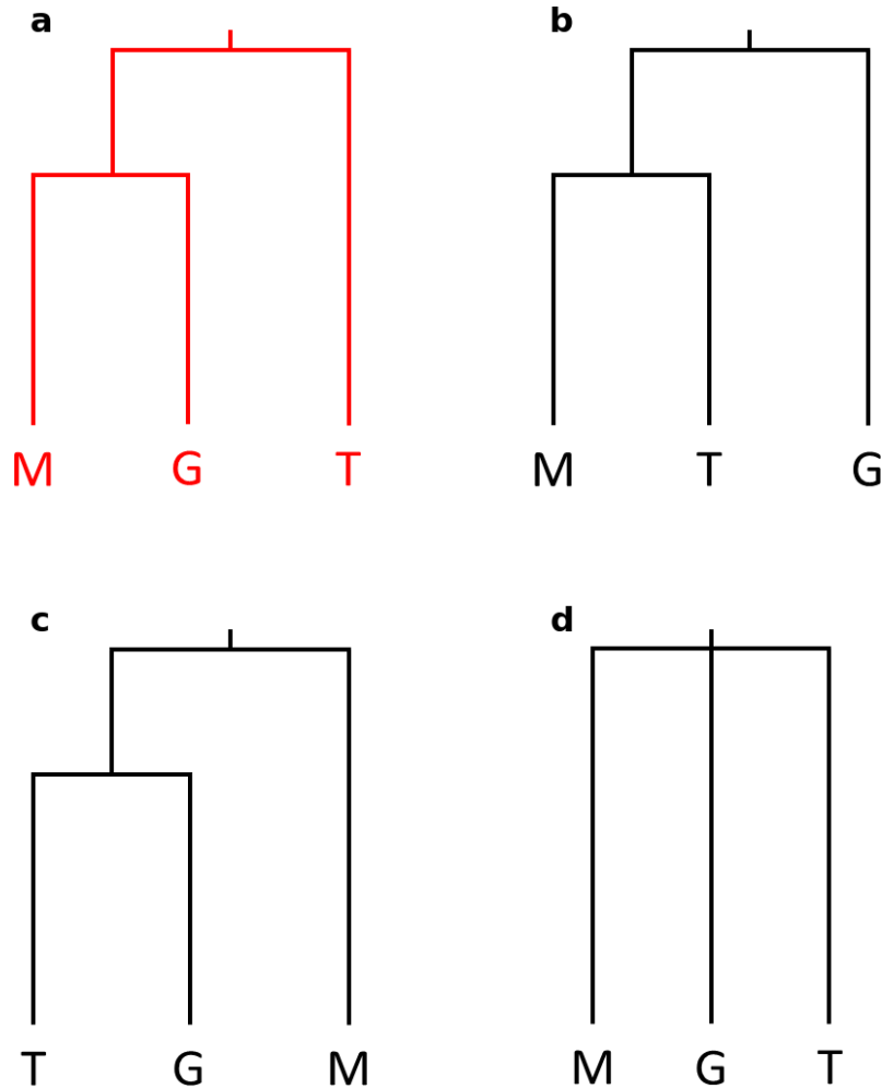
Figure VI-7. Quatre topologies concurrentes sont susceptibles de rendre compte de l'histoire démographique des populations M, G et T. La topologie représentée en rouge ( a ) est la véritable : les populations Maigre (M) et Gras (G) divergent à partir de la même population parentale, tandis que la population Témoin (T) permet d'enraciner l'arbre phylogénétique des populations. Les topologies alternatives considèrent un arbre enraciné avec la population Gras ( b ), Maigre ( c ) ou bien une phylogénie en étoile ( d ).
