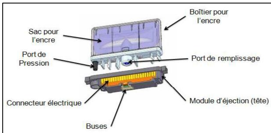
Figure II-12- Cartouche d'impression jet d'encre [115]
