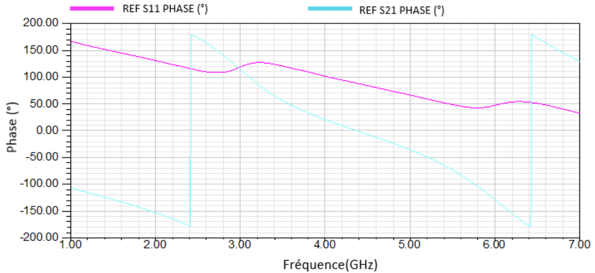
Figure III-22- Simulation des paramètres S en module et en phase du dispositif D1 du résonateur avec couche sensible
