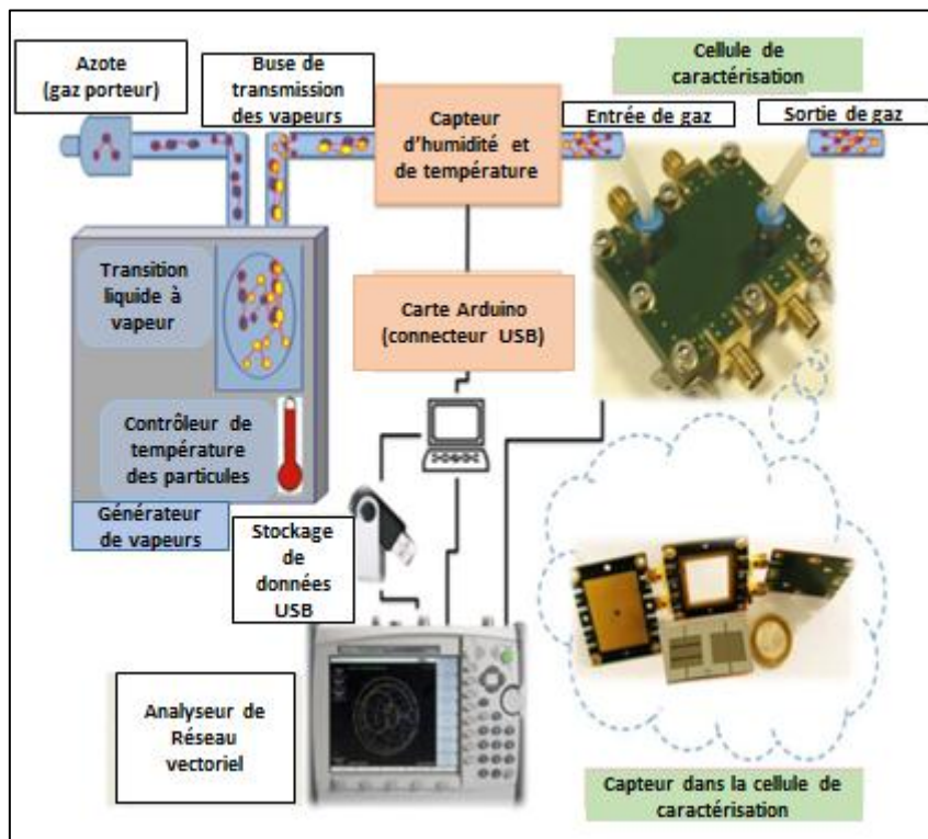
Figure III-36 - Banc de mesure sous gaz [150]
