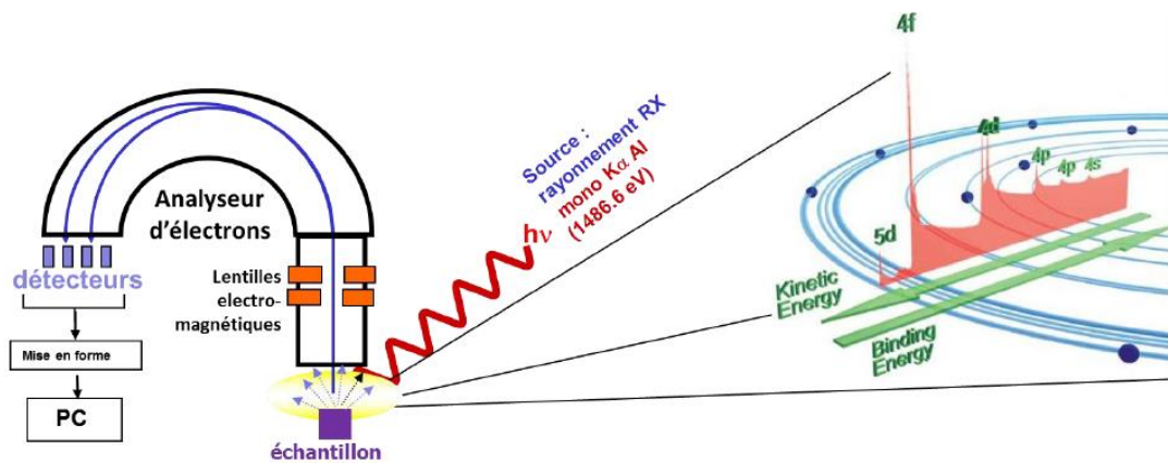
Figure II.8 Schéma de principe d'un spectromètre XPS (Version 05-2015 /JB Ledeuil / IPREM ECP)
