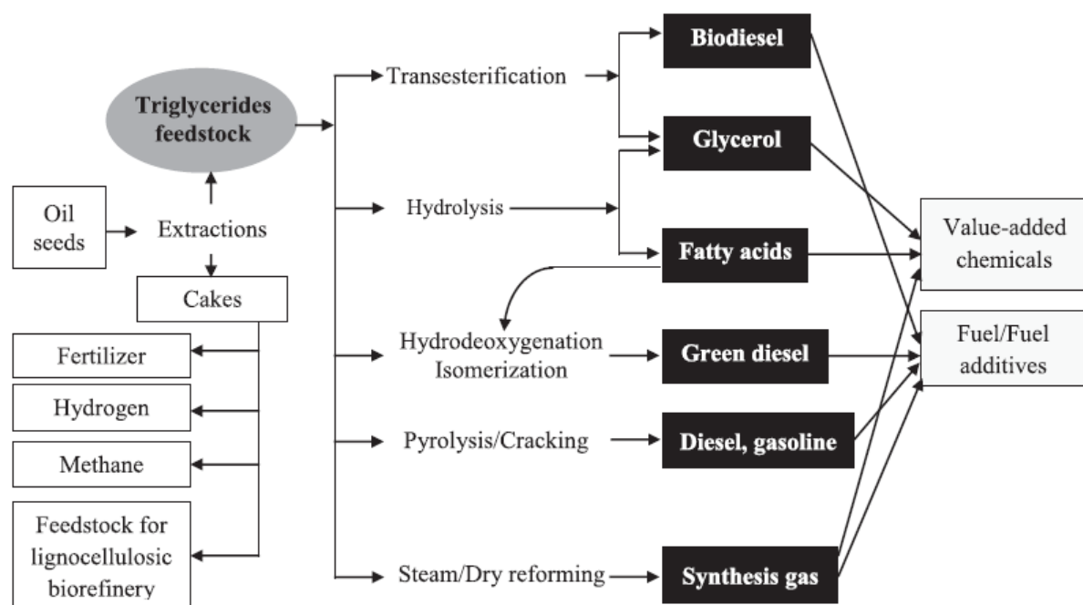
Figure 1-18 : Valorisation d'huiles dans une bioraffinerie [2].
