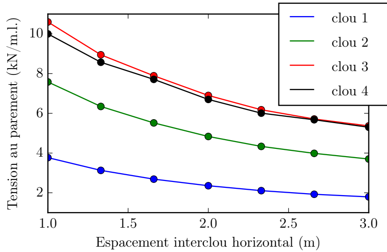
FIGURE 4.37 – Tensions observées au parement par mètre linéaire d'ouvrage dans les clous 1 à 4 en fonction de l'espacement interclou horizontal
