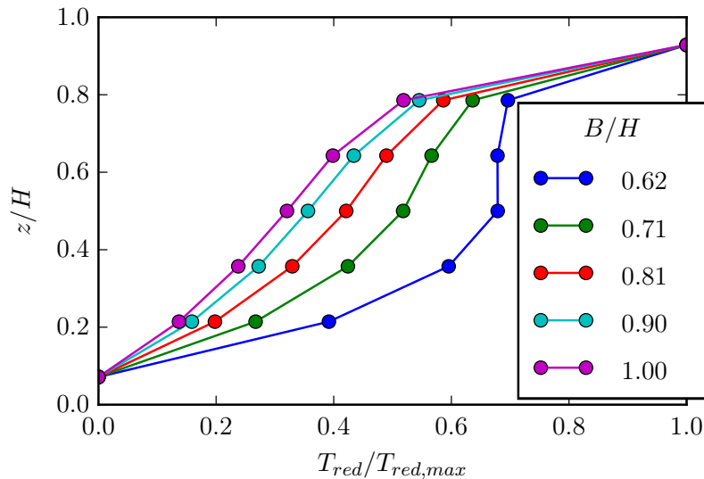
FIGURE 5.1 – Profils d'efforts au parement réduits normalisés calculés pour différents élanagements
