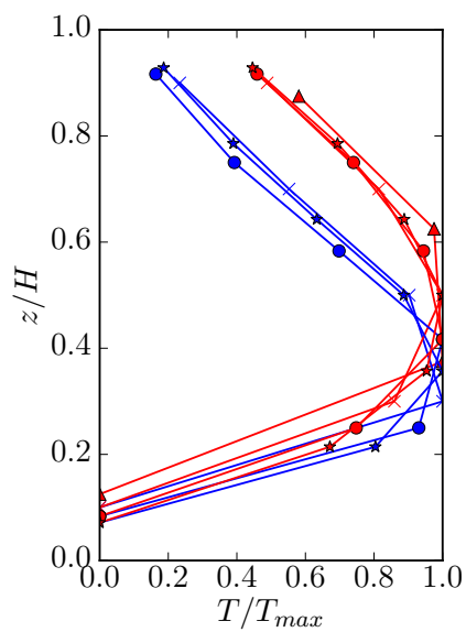
FIGURE 4.31 – Profils normalisés des efforts au parement pour des murs de hauteur variable (6 à 10,5 m) et d'élancements B/H = 1 (en rouge) et B/H \simeq 0,6 (en bleu)
