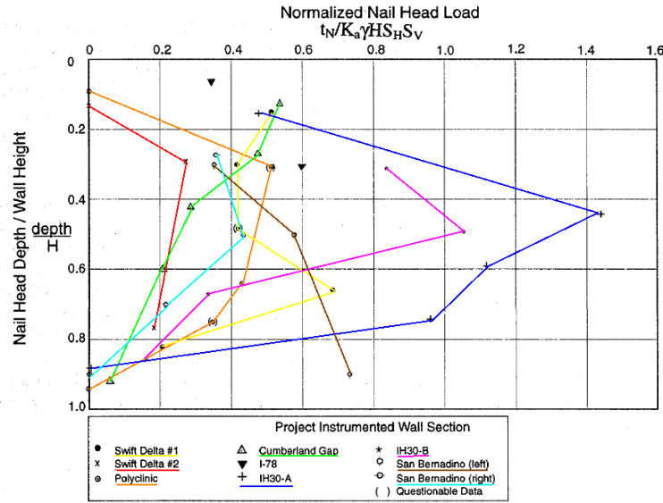
FIGURE 2.3 – Mesures des efforts en tête de clou normalisés par la poussée active pour les différents murs instrumentées par la FHWA (adapté de [14])
