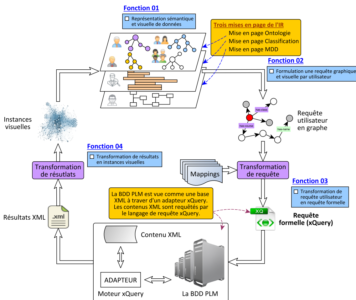
FIGURE 4.10 : Accès sémantique aux données à base de l'ontologie, adapté au domaine du PLM pour Imagerie Biomédicale. Les données BMI gérées par les solutions PLM sont accessibles comme une base XML à travers d'un adapter xQuery (Sriti et Boutinaud 2012). Les utilisateurs formulent leurs requêtes en termes ontologiques sur une interface visuelle et interactive, ces requêtes sont ensuite transformées en requêtes xQuery grâce à un module de transformation et l'ensemble des mappings prédéfinis. Les résultats des requêtes xQuery sont retransformés en instances visuelles dans l'interface de requête.
