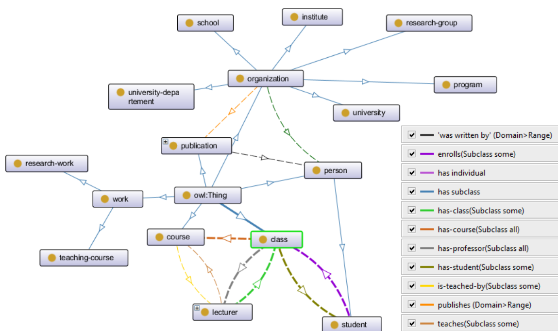
FIGURE 3.3 : Visualisation graphique de toutes les relations sémantiques entre concepts ontologiques.
