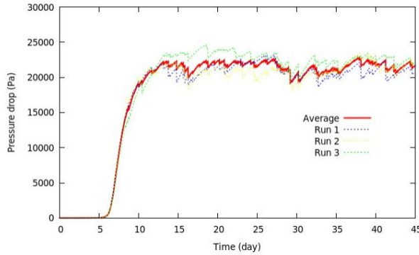
Figure 6.14a: k_{r \max}=80 , k_{r \min}= 80 , \mu_{\max}=5.10^{-5} \text{ s}^{-1} , \Delta t=18000\text{s} , C_s=0.2 \text{ kg/m}^3
