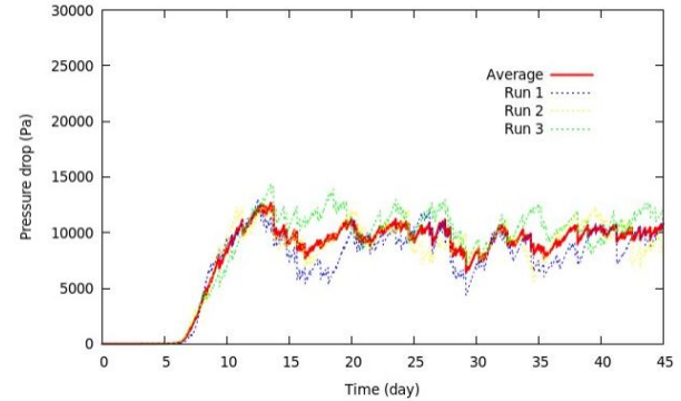
Figure 6.14 b: k_{r \max}=80 , k_{r \min}= 1 , \mu_{\max}=5.10^{-5} \text{ s}^{-1} , \Delta t=18000\text{s} , C_s=0.2 \text{ kg/m}^3
