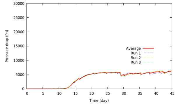
Figure 6.14d: k_{r \max}=500 , k_{r \min}= 80 , \mu_{\max}=5.10^{-5} \text{ s}^{-1} , \Delta t=18000\text{s} , C_s=0.02 \text{ kg/m}^3
