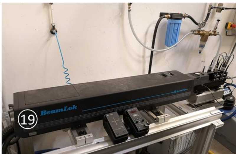
Figure A.3. Photographie de l'installation expérimentale : (15) générateur de vapeur, (16) surchauffeur de vapeur, (17) générateur électrique, (18) générateur de fréquences d'injecteur de gouttes, (19) laser.
