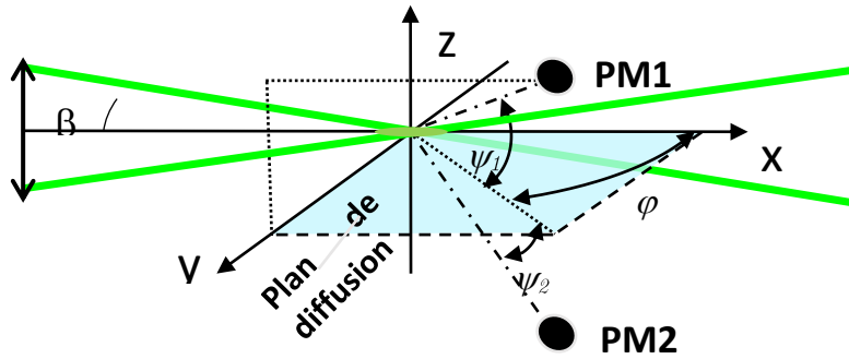
Figure 5.3. Schéma de principe de mesure du PDA.
