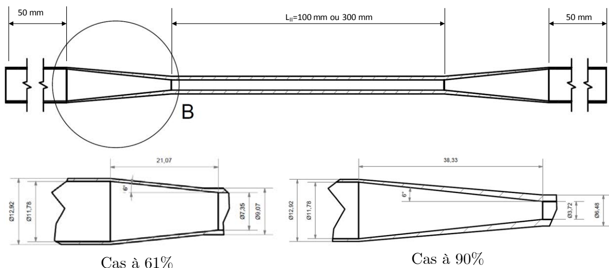
Figure 3.3. Géométrie du venturi, configurations à 61% et à 90%.
