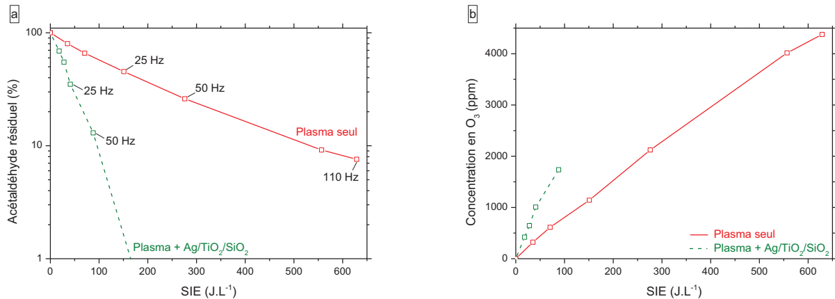
Figure 3-5 : Fraction d'acétaldéhyde résiduel (en %) (a) et concentration en O 3 (en ppm) (b) détectées en sortie de réacteur en fonction de la SIE (en J.L -1 ) lors de la dégradation de l'acétaldéhyde par plasma seul et par plasma-catalyse à température ambiante et pression atmosphérique
