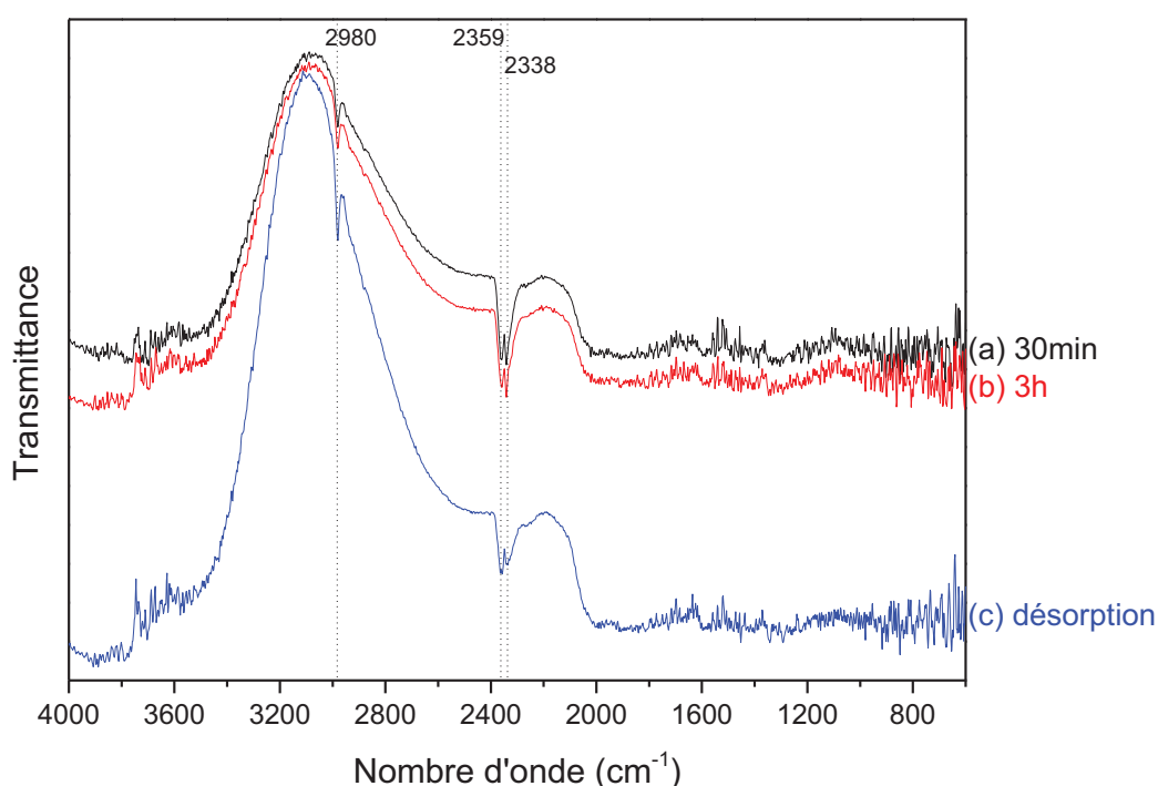
Figure 4-5 : Spectres DRIFTS obtenus après 30 minutes (a) et 3 heures (b) d'adsorption du mélange \text{CO}_2 (250 ppmC) dans \text{N}_2/\text{O}_2 (20 %) sur \text{Ag}/\text{TiO}_2/\text{SiO}_2 , et après 45 minutes de désorption sous \text{N}_2 pur (c) à température ambiante et pression atmosphérique
