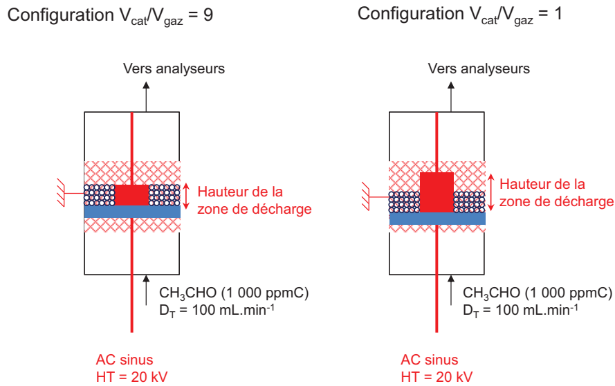
Figure 3-18 : Schéma du dispositif en configuration V_{cat}/V_{gaz} = 9 et V_{cat}/V_{gaz} = 1
