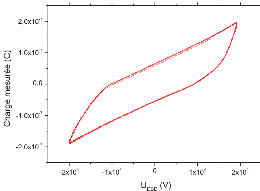
Figure 2-7 : Exemple d'une courbe de Lissajous obtenue lors de la dégradation de \text{CH}_3\text{CHO} (1 000 ppmC) dans \text{N}_2/\text{O}_2 (20 %) par le procédé plasma seul (HV = 20 kV, f = 25 Hz, D_T = 100 mL.min -1 , C_{\text{mesure}} = 8 nF)
