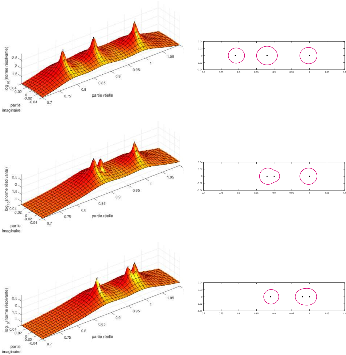
FIGURE 5.3 – Représentation de la norme euclidienne de la résolvente pour une matrice stochastique P de dimension 3 et du contour de la norme de la résolvente. Les trois comportements discutés sont illustrés.
