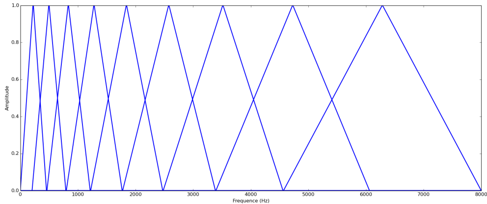
FIGURE 2.6 – Réponse fréquentielle d’une banque de 10 filtres suivant l’échelle perceptuelle Mel sur l’espace fréquentiel [0-8000Hz].
