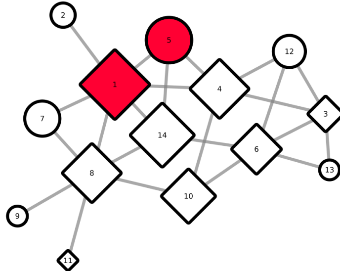
Figure 7.1 – Illustration de la centralité de proximité : exemple du réseau d’interactions sociales d’une colonie de babouins. Les losanges représentent les individus femelles, et les ronds les individus mâles. Les arêtes représentent les interactions sociales (essentiellement les événements de toilettage mutuels). La taille des nœuds est proportionnelle à la closeness . Les nœuds rouges représentent le mâle leader et la femelle dominante du groupe. Les numéros des nœuds correspondent aux identifiants des individus.
