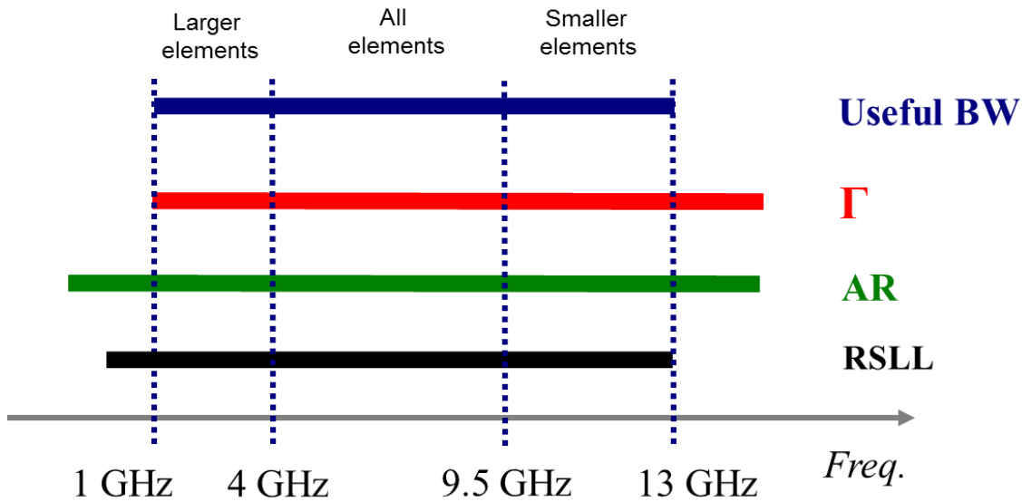
Figure 4 Les barres correspondent aux définitions de bande passante ci-après. En rouge nous avons la barre qui correspond au coefficient de réflexion, en vert le rapport axiale et en noir le niveau des lobes secondaires relative. La bande passante utile est l'intersection de ces trois bandes passantes.
