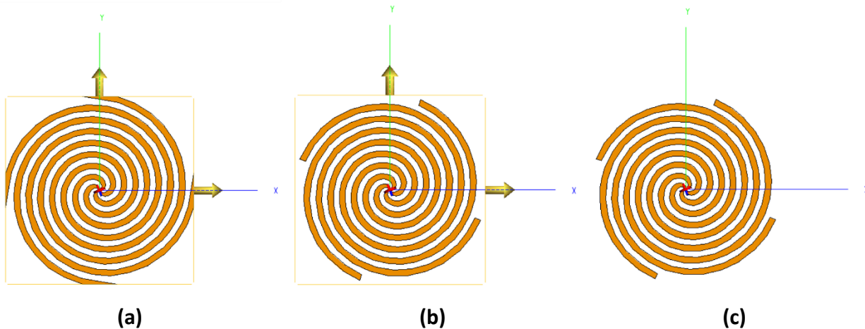
Figure 6 Modèles FEKO correspondant, de gauche à droite, au réseau infini de spirales à quatre bras connectés, au réseau infini de spirales à quatre bras non connectés et à une seule spirale à quatre bras. Les spirales ont un rayon égal à 2.4 cm.
