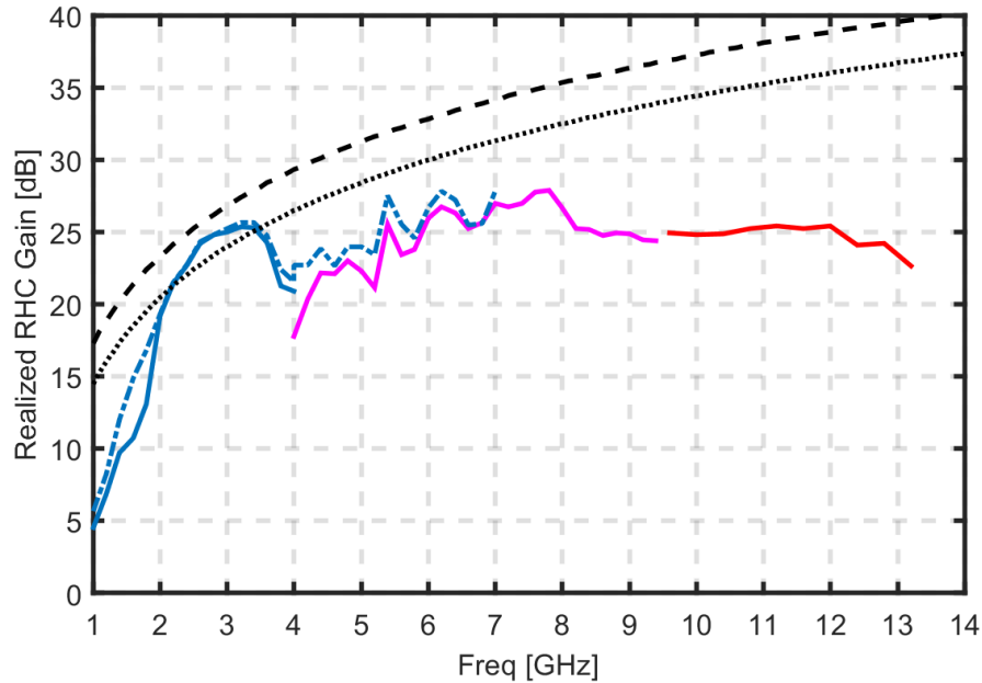
Figure 5 Courbes de gain réalisé à “broadside” pour le réseau d’anneaux concentriques de la section 2.3.3 (ligne bleu tireté) et pour le réseau d’anneaux concentriques avec WAVES de la section 2.4.1 avec que les éléments grands allumés (bleu), les éléments grands et petits allumés en même temps (magenta) et seulement les éléments petits allumés (rouge). Superposé nous avons le gain surfacique maximal correspondant au cercle de rayon de 35 cm (surface de 0.38 m 2 ) auquel les réseaux sont circonscrits (ligne noir tireté) aussi que celui correspondant à la surface occupé par les cavités des réseaux d’anneaux concentriques avec et sans WAVES, qui sont égales à 0.2 m 2 dans les deux cas (ligne noir pointillé).
