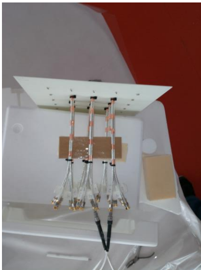
Figure 8 Mesure des paramètres S du prototype du réseau de spirales non complémentaires à quatre bras connectés.
