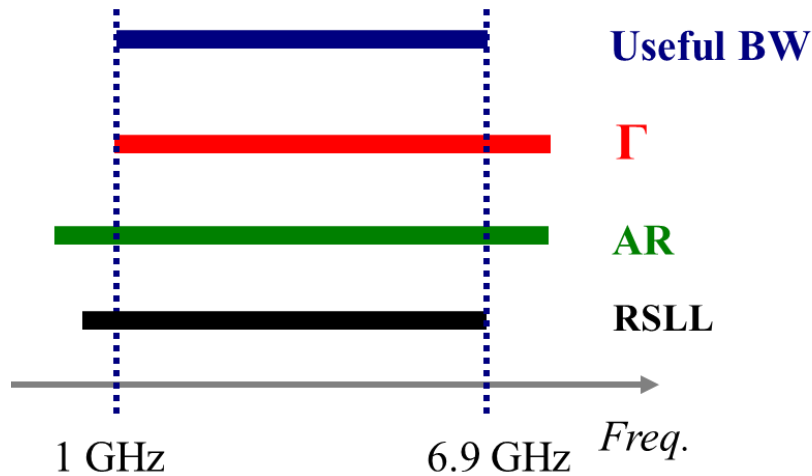
Figure 2 Les barres correspondent aux définitions de bande passante ci-après. En rouge nous avons la barre qui correspond au coefficient de réflexion, en vert le rapport axial et en noir le niveau des lobes secondaires relative. La bande passante utile est l'intersection de ces trois bandes passantes.
