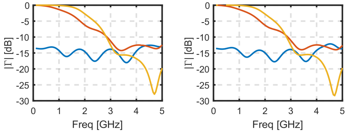
Figure 7 Simulation FEKO du réseau infini de spirales à quatre bras connectés (bleu), du réseau infini de spirales à quatre bras non connectés (rouge) et de la spirale à quatre bras seule (jaune). Les courbes à gauche montrent la polarisation principale (mode 1) et les courbes à droite montrent la polarisation secondaire (mode -1). Les courbes en tireté noir montrent le gain surfacique maximal correspondant à la région enfermée par les limites périodiques moins 3 dB pour compenser le fait que les antennes rayonnent des deux côtés.
