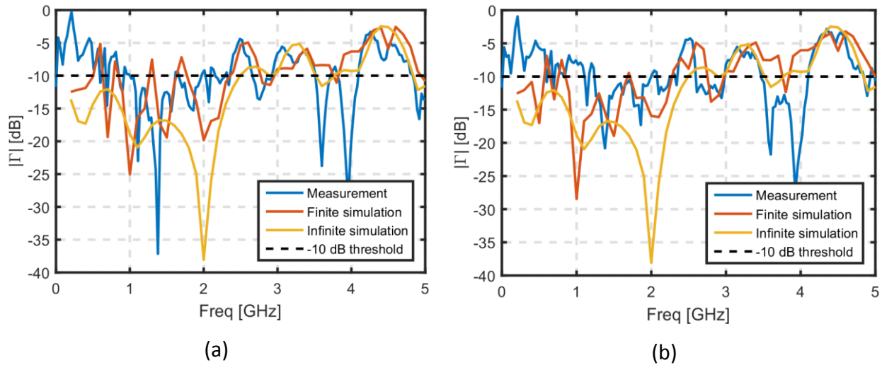
Figure 9 Coefficient de réflexion du réseau prototype, de la simulation FEKO du réseau de 3x3 spirales non complémentaires à quatre bras connectés avec une couche d'éléments adaptés par des résistances de 100 \Omega et de la simulation FEKO du réseau infini de spirales non complémentaires à quatre bras connectés. En (a) nous avons le réseau avec polarisation circulaire main droite (mode 1) et en (b) nous avons le réseau avec polarisation circulaire main gauche (mode-1).
