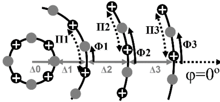
Figure 1 Réseau d'anneaux concentriques : les cercles remplis et avec des croix représentent, respectivement, les spirales polarisés main gauche et main droite. Les spirales sont intercalées, ce qui rend le réseau lacunaire, et alors des lobes secondaires hauts (« lobes de réseau ») apparaissent dans la zone visible de rayonnement. Les anneaux concentriques peuvent avoir les rayons et rotations relatives optimisés pour réduire ces lobes et alors réduire le niveau de lobes secondaires relative à hautes fréquences.
