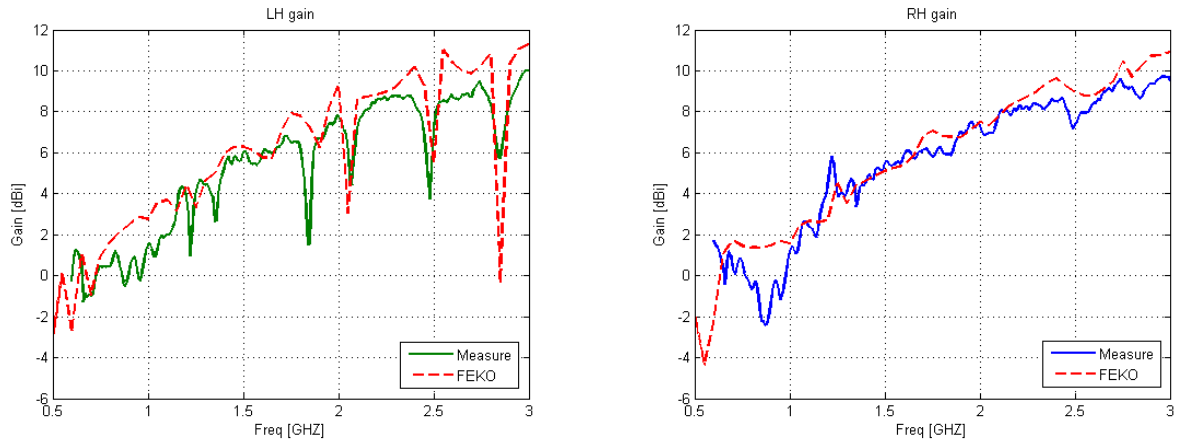
Figure 10 Gain de la composante à polarisation circulaire main droite et main gauche du réseau prototype et de la simulation FEKO du réseau de 3x3 spirales non complémentaires à quatre bras connectés avec une couche d'éléments adaptés par des résistances de 100 \Omega .
