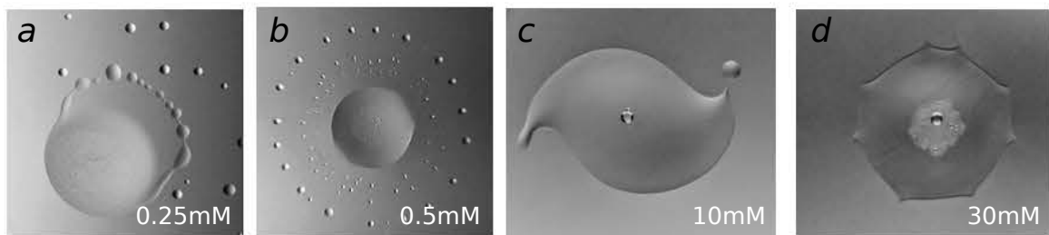
Figure 2.9: Différents régimes controlés par la concentration de CTAB. a: Etallement. b: Pulsation. c: Rotation. d: goutte en forme polygonale
