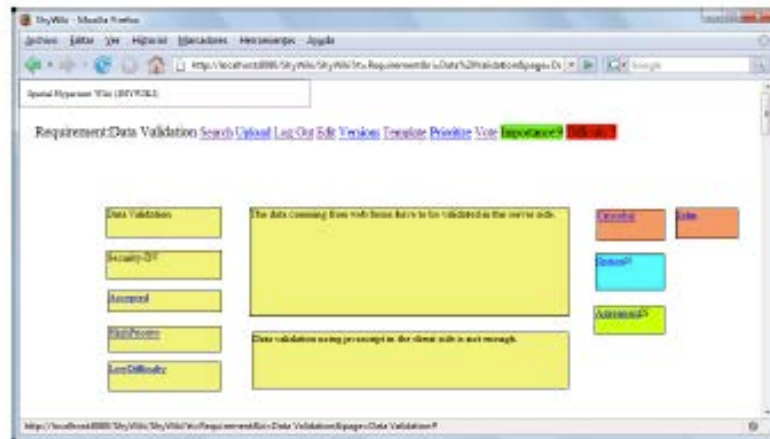
Figure 68: ShyWiki, un wiki comme support au brainstorming entre parties prenantes (Solis et Ali 2010)
