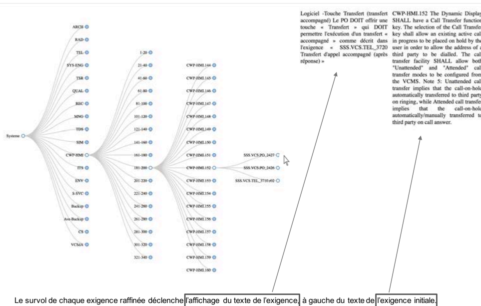
Figure 98: affichage des exigences raffinées par survol successif d'un arbre dépliant
