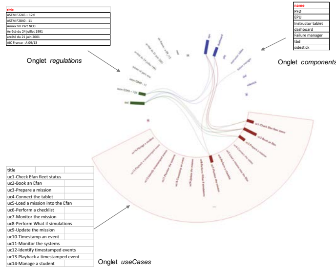
Figure 121: construction du chord diagram à partir d'onglets du fichier Excel
