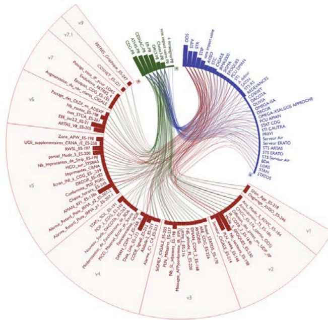
Figure 108: la visualisation de chord diagram pour voir les composants système (en bleu) implémentant les évolutions (en rouge) selon les sites opérationnels (en vert)
