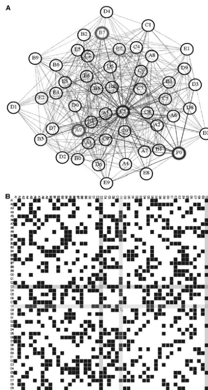
Figure 95: deux visualisations du même graphe (50 noeuds, 400 arcs): diagramme de réseau et matrice (Ghoniem, Fekete, et Castagliola 2005)
