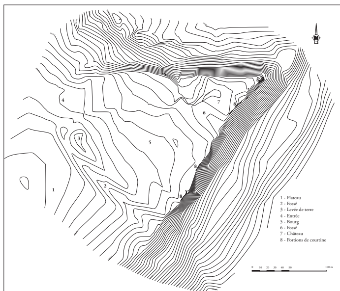
Fig. 1 – Relevé topographique du bourg castral et du château de Châtenois, XI e -XVII e siècles, Vosges (relevé Jérôme Balay, Gérard Giuliano, Charles Kraemer).
