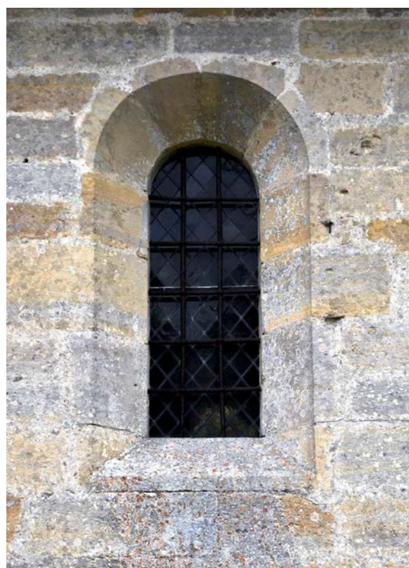
Fig. 26 – Arc composé de quatre voussoirs, sans clef d'arc, église de Couvonges, 55 (cliché Cédric Moulis).
