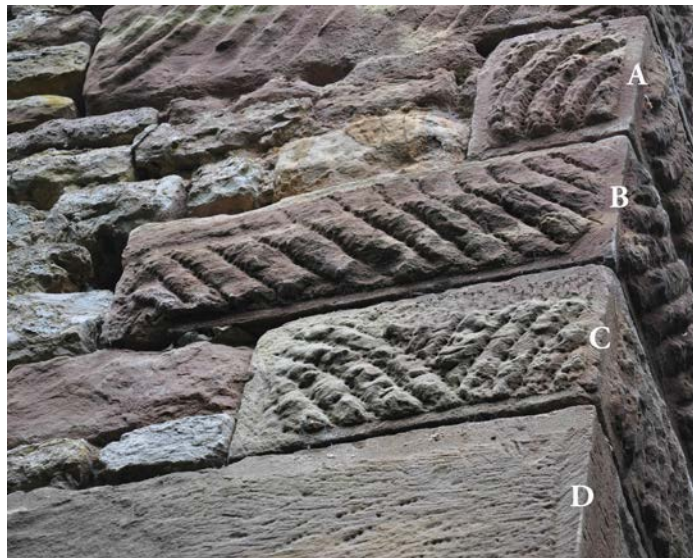
Fig. 17 – La chaîne d'angle du château de Romont (88) montre bien le recul du travail de taille plus on monte dans l'élévation. Cela permet de dérouler dans l'ordre chronologique les différentes étapes de la taille de ces pierres, de A à D (cliché Cédric Moulis).
