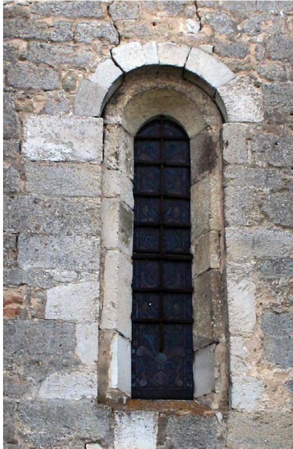
Fig. 27 – Sur le chevet de Choloy (54), l'arc monolithe sert de support au montage de l'arc en extrados, qui agit ensuite comme un arc de décharge (cliché Marion Subts).
