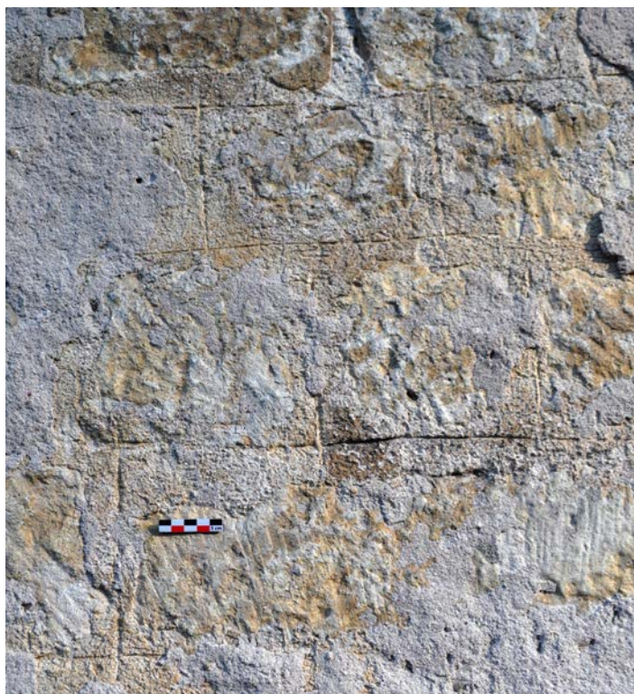
Fig. 16 – Décor de joints fins tirés au fer sur un parement de pierres équarries, église de Vandœuvre, 54 (cliché Cédric Moulis).
