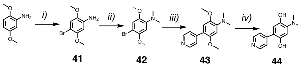
Schéma 18 : Stratégie synthétique pour la préparation de 44 : i) \text{Br}_2 , \text{CH}_2\text{Cl}_2 , 0^\circ\text{C} à ta, 12 heures; ii) \text{NaBH}_4 , \text{CH}_2\text{O} , THF, 0^\circ\text{C} à ta, 12 heures; iii) acide 4-pyridinilboronique, \text{K}_2\text{CO}_3 , \text{Pd}(\text{PPh}_3)_4 , THF/MeOH/ \text{H}_2\text{O} , 65^\circ\text{C} , 4 jours; iv) \text{BBr}_3 , \text{CH}_2\text{Cl}_2 sec, -78^\circ\text{C} à ta, 24 heures.
