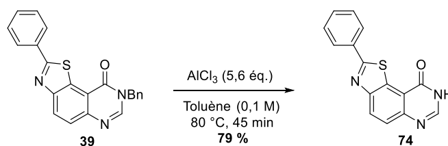
Schéma II-53 : déprotection du composé mono-arylé 39 en présence du chlorure d'aluminium.
