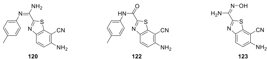
Figure IV-3 : Structures des composés 120 , 122 et 123 .
