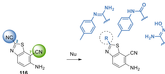
Schéma 27 : Etude de la régiosélectivité du 6-aminobenzo[d]thiazole-2,7-dicarbonitrile 116 .
