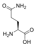
L-Glutamine (Gln)
