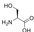
L-Sérine (Ser)
