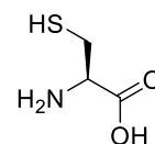
L-Cystéine (Cys)
