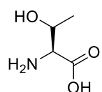
L-Thréonine (Thr)
