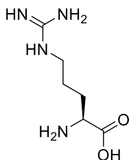
L-Arginine (Arg)
