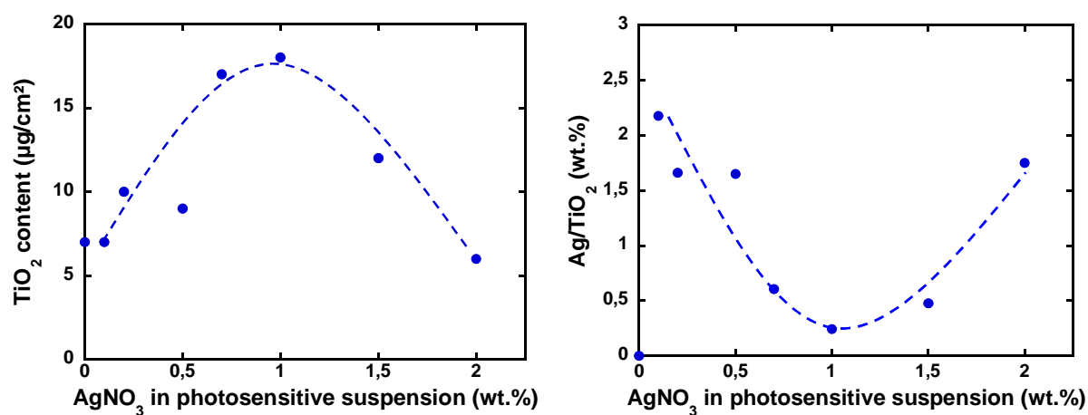
Fig. 12: Teneur en TiO 2 (gauche) et rapport massique Ag/TiO 2 (droite) des films hybrides PEI/PSS/(Ag-TiO 2 ) en fonction de la concentration en AgNO 3 dans la suspension photosensible.
