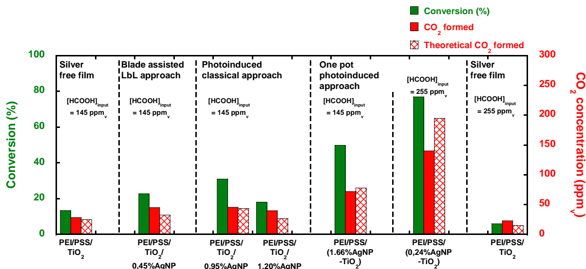
Fig. 15: Comparaison des performances photocatalytiques des films PEI/PSS/(Ag-TiO 2 ) préparés selon les 3 différentes méthodes. Conditions expérimentales : débit total = 20 mL/min, UV-A (2.5 mW/cm 2 ), substrat modèle de 36 cm 2 .
