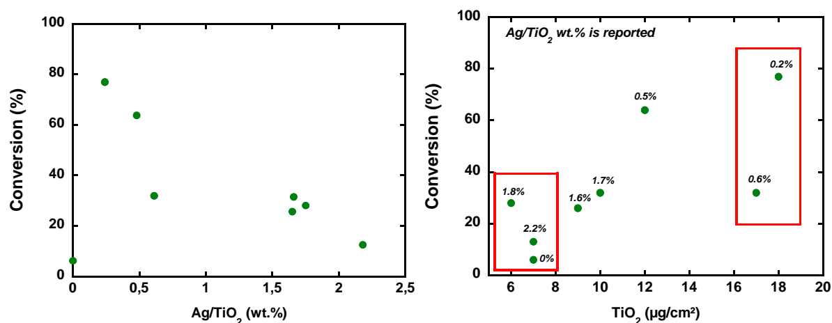
Fig. 13: Résultats des tests photocatalytiques de dégradation de HCOOH en phase gazeuse (gauche) en fonction du rapport massique Ag/TiO 2 , et (droite) en fonction de la teneur en TiO 2 dans les films PEI/PSS/(Ag-TiO 2 ). Conditions expérimentales : [HCOOH] = 255 ppm v , débit total = 20 mL/min, UV-A (2.5 mW/cm 2 ), substrat modèle de 36 cm 2 .
