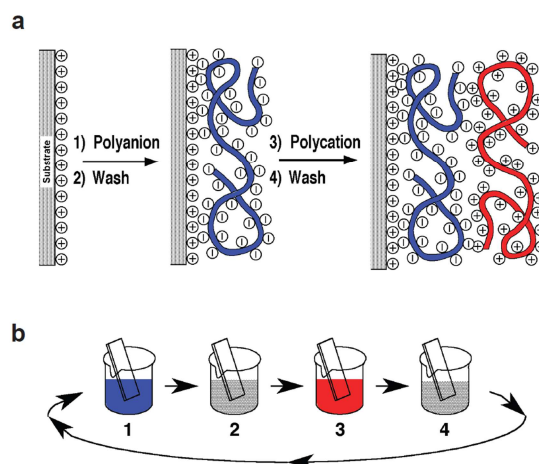
Fig. 2: (a) Schématisation de la construction d'un film multicouche de polyelectrolytes par la technique du LbL sur une surface plane. (b) Construction des films LbL par la méthode de trempage. Les étapes intermédiaires de rinçage dans de l'eau, permettent la surcompensation des charges et d'enlever l'excès de matériaux non adsorbé. La versatilité de cette technique lui permet d'utiliser différents types de matériaux, tels que des nanoparticules, et d'être appliquée sur des surfaces de géométries variées [17], [18].
