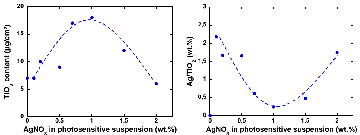
Fig. 12: Teneur en TiO 2 (gauche) et rapport massique Ag/TiO 2 (droite) des films hybrides PEI/PSS/(Ag-TiO 2 ) en fonction de la concentration en AgNO 3 dans la suspension photosensible.
