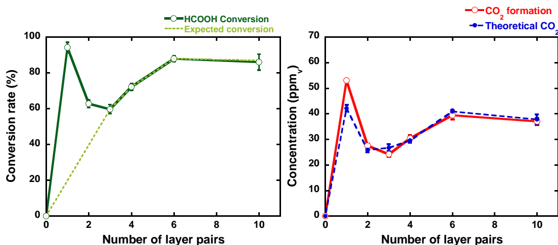
Fig. 7: Dégradation de l'acide formique et minéralisation en CO 2 sous UV-A par des films PEI/(PSS/TiO 2 ) n . Conditions expérimentales : [HCOOH] = 45 ppm vol , débit total = 20 mL/min, UV-A (2.5 mW/cm 2 ), substrat modèle de 36 cm 2 (8 cm x 4.5 cm). A gauche : conversion d'acide formique en fonction du nombre de paires de couches. La courbe en pointillé montre un comportement classique de la dégradation d'un polluant en fonction de la concentration en TiO 2 ; la courbe pleine représente le comportement observé lors des tests photocatalytiques. A droite : formation de CO 2 montrant le même comportement que la conversion de l'acide formique ; la courbe en pointillé représente la concentration en CO 2 correspondant à sa formation stoechiométrique par rapport à la conversion de l'acide formique.
