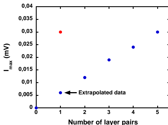
Fig. 14: Valeur de l'intensité maximale I_{max} caractéristique dérivée des mesures de TRMC sur les films PEI/(PSS/TiO 2 ) n (•) et PEI/PSS/(Ag-TiO 2 ) (•). Irradiation laser à 350 nm.
