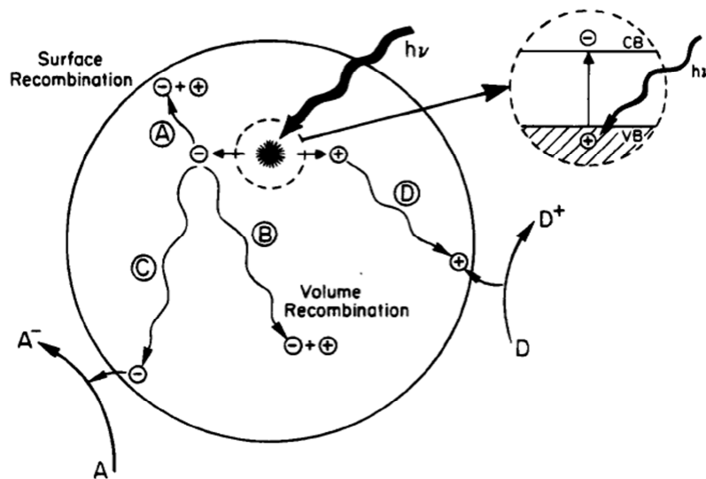
Fig. 1: Principe simplifié d'une réaction photocatalytique avec un matériau semi-conducteur sous irradiation h\nu [12].
