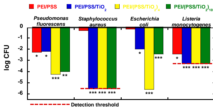
Fig. 18: Tests antibactériens des films multicouches PEI/(PSS/TiO 2 ) n . Bactéries testées : Pseudomonas fluorescens , Staphylococcus aureus , Escherichia Coli K12 et Listeria monocytogenes , UV-A (2.5 mW/cm 2 ), temps d’irradiation = 3 h, textiles en fibre de polyester de 2 cm 2 . Tests effectués selon la norme BS ISO 27447. p : p-value ; (*) p < 0.05, (**) p < 0.001, (***) p < 0.0001
