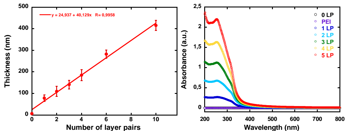
Fig. 5: Suivi de la construction des films PEI/(PSS/TiO 2 ) n (à gauche) par ellipsométrie pour des films construits sur wafer de silicium, (à droite) par spectrophotométrie UV-Visible pour des films construits sur des lamelles de quartz.
