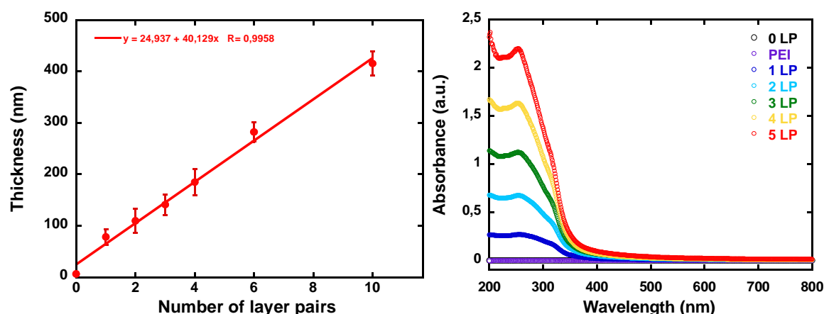
Fig. 5: Suivi de la construction des films \text{PEI}/(\text{PSS}/\text{TiO}_2)_n (à gauche) par ellipsométrie pour des films construits sur wafer de silicium, (à droite) par spectrophotométrie UV-Visible pour des films construits sur des lamelles de quartz.
