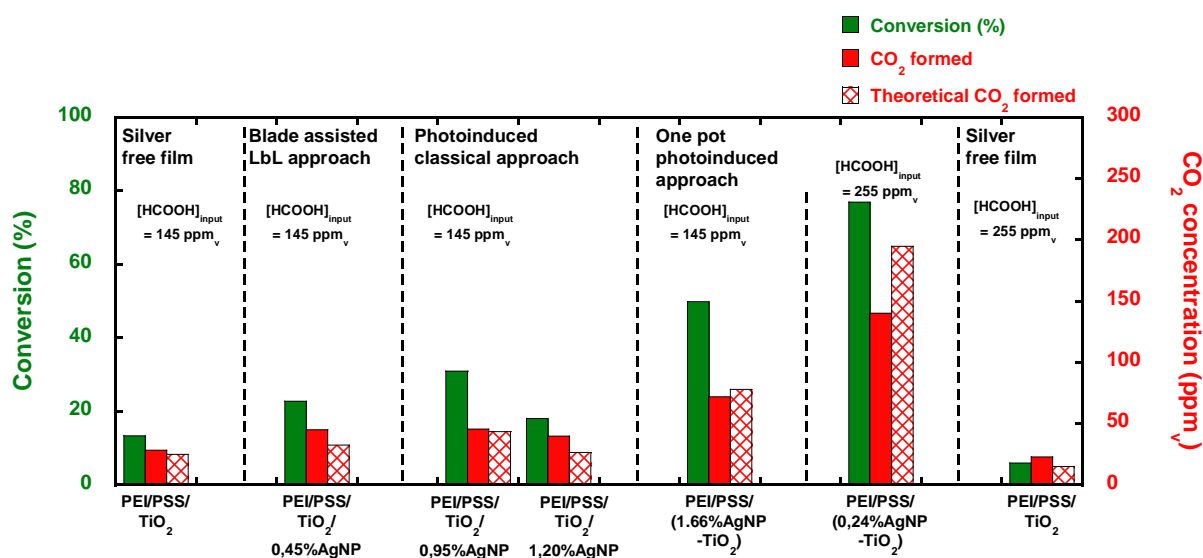
Fig. 15: Comparaison des performances photocatalytiques des films PEI/PSS/(Ag-TiO 2 ) préparés selon les 3 différentes méthodes. Conditions expérimentales : débit total = 20 mL/min, UV-A (2.5 mW/cm 2 ), substrat modèle de 36 cm 2 .
