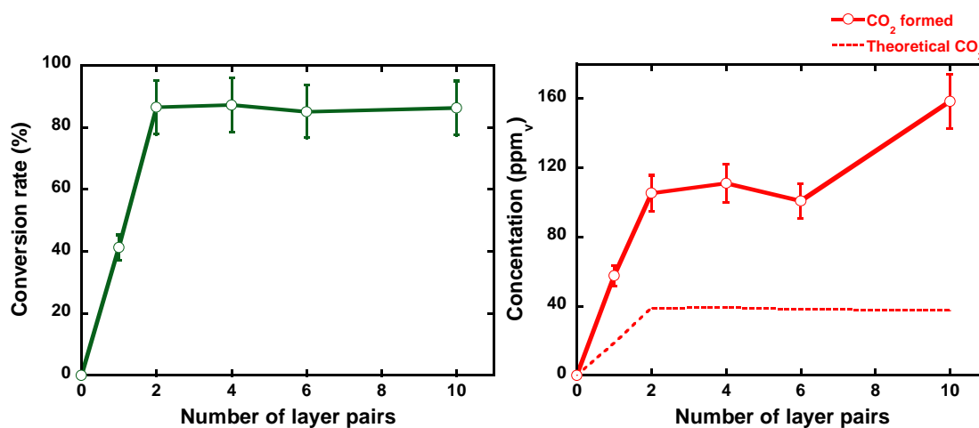
Fig. 17: Test photocatalytiques de dégradation de HCOOH en phase gazeuse pour les films PEI/(PSS/TiO 2 ) n construits sur textiles polyester. (A gauche) Conversion d'acide formique en fonction du nombre de paires de couches. (A droite) Formation de CO 2 ; la courbe en pointillé représente la concentration en CO 2 correspondant à sa formation stoechiométrique par rapport à la conversion de l'acide formique. Conditions expérimentales : [HCOOH] = 45 ppm vol , débit total = 20 mL/min, UV-A (2.5 mW/cm 2 ), textiles en fibre de polyester de 36 cm 2 .
