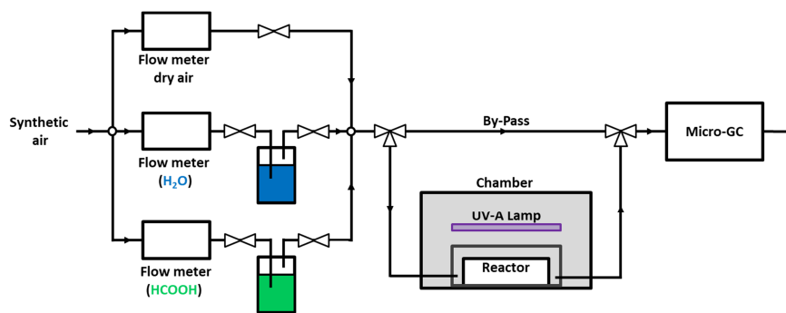
Fig. 4: Schéma du montage du test photocatalytique pour la dégradation de l'acide formique en phase gazeuse.
