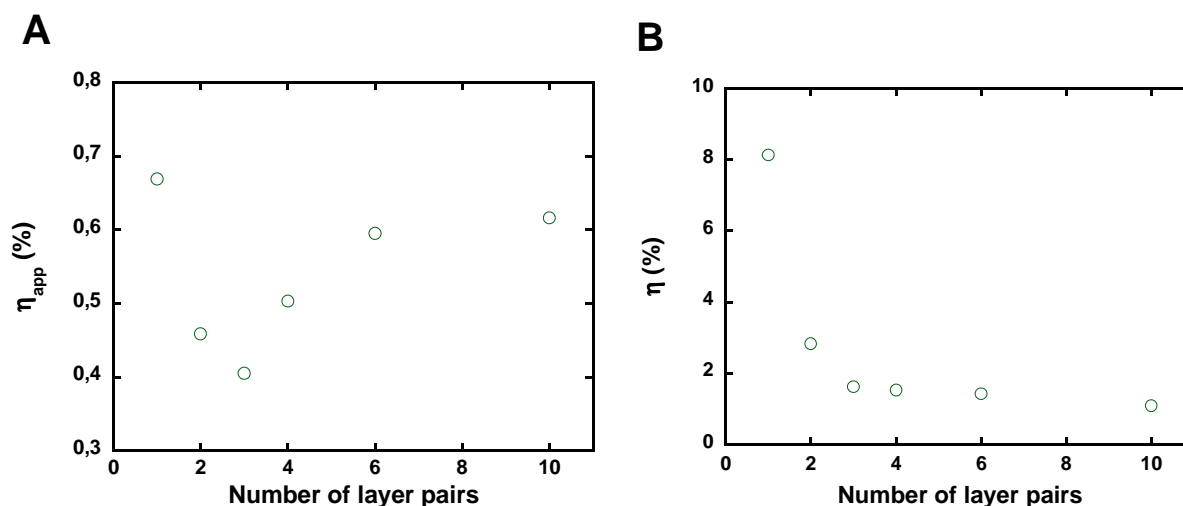
Fig. 8: Rendement quantique apparent (A) et efficace (B) des films PEI/(PSS/TiO 2 ) n en fonction du nombre de paires de couches. Le rendement quantique apparent se réfère à la quantité de photons reçue par le film, tandis que le rendement quantique efficace fait référence à la quantité de photons absorbée par le film.
