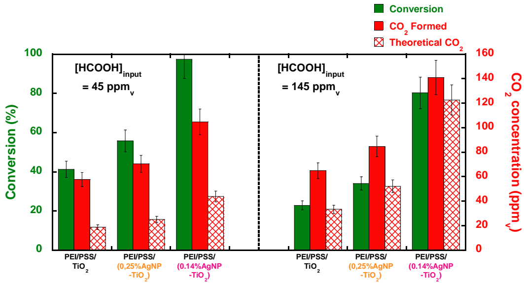
Fig. 19: Test photocatalytiques pour la dégradation de HCOOH en phase gazeuse pour les films PEI/PSS/(Ag-TiO 2 ) construits sur textiles. Conditions expérimentales : [HCOOH] = 45 ppm v (à gauche), 145 ppm v (à droite) , débit total = 20 mL/min, UV-A (2.5 mW/cm 2 ), textiles en fibre de polyester de 36 cm 2 .
