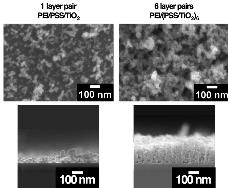
Fig. 6: Caractérisation par microscopie électronique à balayage des films multicouches contenant une et 6 paires de couches. Les images du bas représentent une coupe transverse des échantillons.
