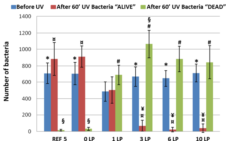
Fig. 9: Tests antibactériens des films multicouches PEI/(PSS/TiO 2 ) n . Bactéries testées : Escherichia Coli , UV-A (2.5 mW/cm 2 ), temps d'irradiation = 60 min, wafer de silicium de 2 cm 2 . Le nombre de bactéries ( Escherichia coli SCC1) dites « ALIVE » et « DEAD » est déterminé par microscopie confocale. « REF 5 » représente un film multicouches comportant 9 paires de couches de poly(styrène sulfonate), PSS, et de poly(diallyldiméthylammonium), PDDA, (PEI/(PSS/PDDA)) 9 . (*) significativement différent de « 1LP before UV » (p < 0.05) ; (⌘) significativement différent de « 1 LP after UV (ALIVE) » (p < 0.05) ; (¥) significativement différent de « 0 LP, 1 LP et REF 5 after UV (ALIVE) » (p < 0.05) ; (#) significativement différent de « 0 LP after UV (DEAD) » (p < 0.05) ; (§) significativement différent de « 1 LP after UV (DEAD) » (p < 0.05).
