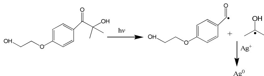
Fig. 10: Photo-clivage du chromophore Irgacure 2959 et réduction des cations \text{Ag}^+ lors de la synthèse photoinduite des nanoparticules d'argent.
