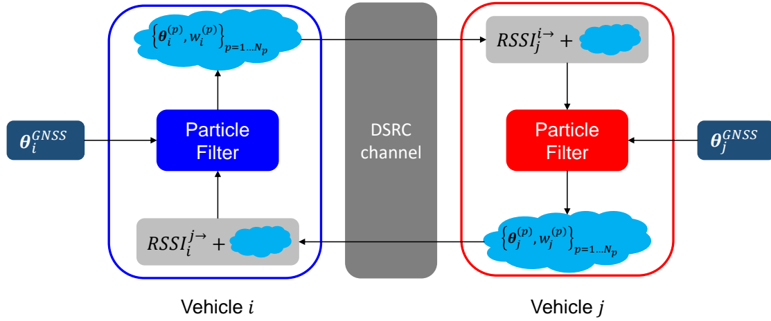
Figure 9.14: Flot de données dans un contexte de fusion coopérative à base de filtre particulaire entre deux véhicules où, pour le véhicule i , \theta_i^{GNSS} , RSSI_i^{j \rightarrow} et \{\theta_i^{(p)}, w_i^{(p)}\}_{p=1 \dots N_p} représentent respectivement l'estimation GNSS, la mesure RSSI réalisée à partir du message CAM reçu de la part de j , et le nuage de N_p particules et représenté par \theta_i^{(p)} et w_i^{(p)} , respectivement les états et poids associés. Le canal de communication ITS-G5 (DSRC) est sujet à des limitations imposées par le standard (ex. taille maximale des messages: 300 – 800 octets, capacité maximale: 6 Mbps, contrôle décentralisé de congestion imposant une réduction à 2 Hz du taux d'émission des messages en cas de de surcharge avérée du réseau...).
