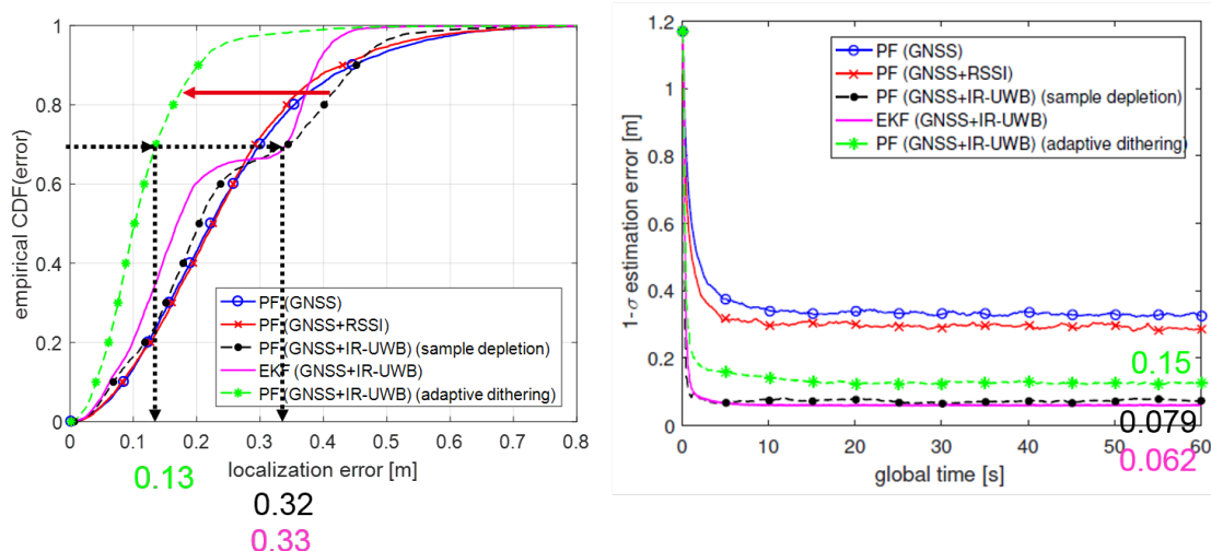
Figure 9.19: CDF empirique de l'erreur de positionnement issue de la fusion ITS-G5/GNSS/IR-UWB et erreurs caractéristiques effectives à 1\text{-}\sigma (c.-à-d. à \text{CDF}=68\% ), pour différentes stratégies de filtrage (gauche) et évolution de l'erreur à 1\text{-}\sigma perçue au niveau des filtres, en fonction du temps (droite).
