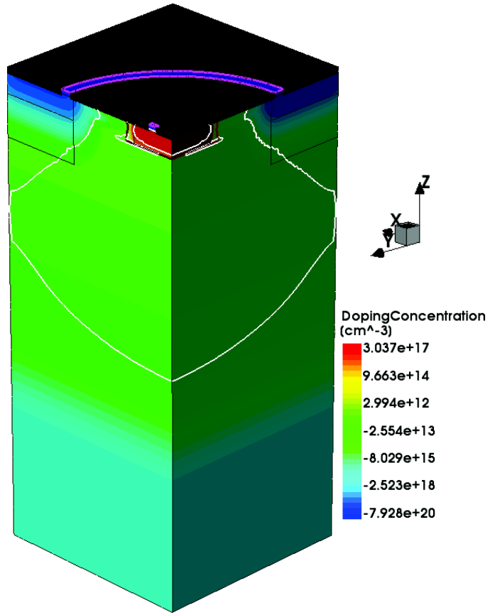
Figure 5: Structure réaliste du pixel PIPPER-2 étudié simulé par éléments finis polarisé à 20 V. La zone désertée est délimitée par la ligne blanche
