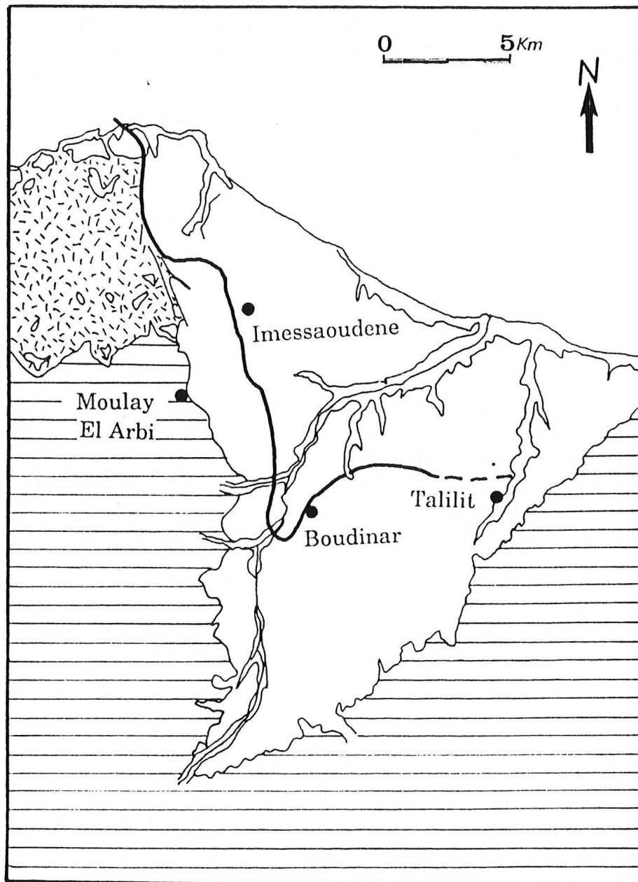
Fig . 55 - Limites du rivages de la mer pliocène (en trait gras) (d'après El Kharim, 1990)
