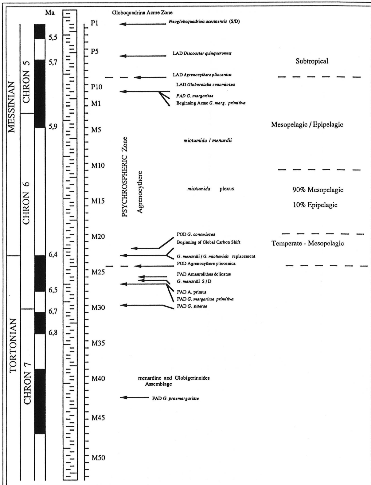
Fig. 36- Succession des bio- événements et changement de populations de foraminifères planctonique à la limite Tortonien-Messinien dans la région de Rabat (d'après Benson et al. , 1990)
