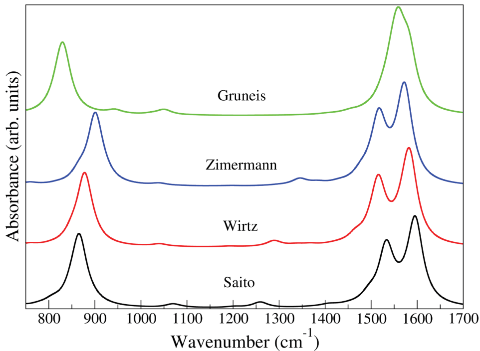
FIGURE 6.4 – Spectres d'absorption infrarouge du nanotube (11,0) calculés selon le modèle de Saito, Grüneis, Wirtz et Zimermann.
