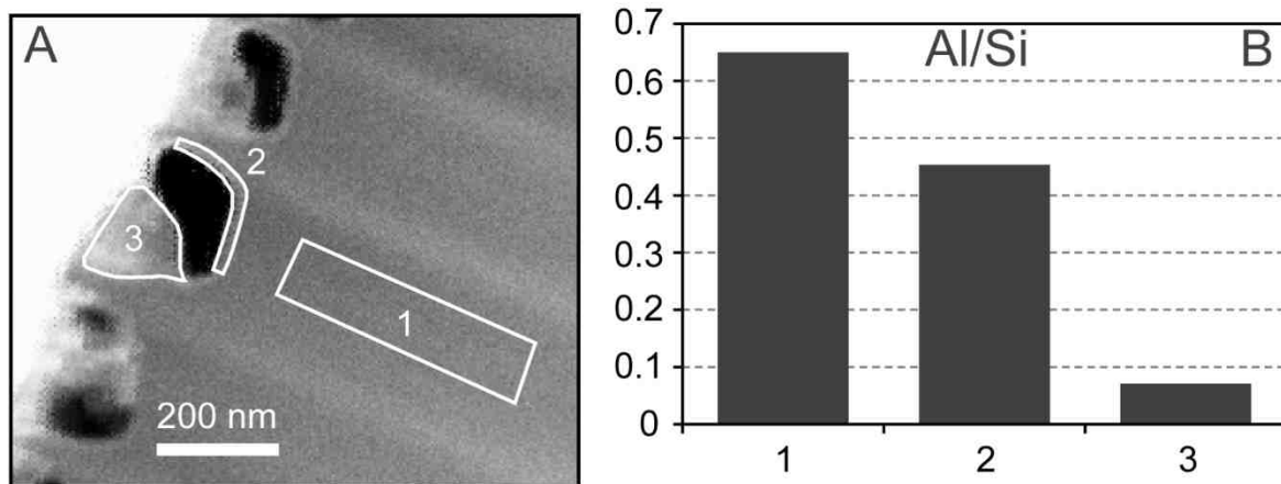
Figure IV.10 : Image STEM d'un échantillon de labradorite ayant réagi à \text{pH} = 2,5 dans une solution d'HCl à 80^\circ\text{C} à saturation vis-à-vis de la silice amorphe pendant 20 jours. Les rapports Al/Si basés sur les valeurs de pourcentages atomiques déterminés sur la labradorite saine (1), la portion de couche au contact de la labradorite saine (2) et la portion de couche rétractée au séchage (3) sont présentés en (B).
