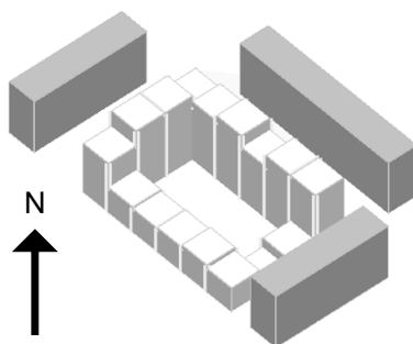
Figure I.22 – Solution permettant de minimiser les besoins de chauffage d'un îlot urbain (variables : hauteur des bâtiments) - d'après Vermeulen, 2014 [15].
