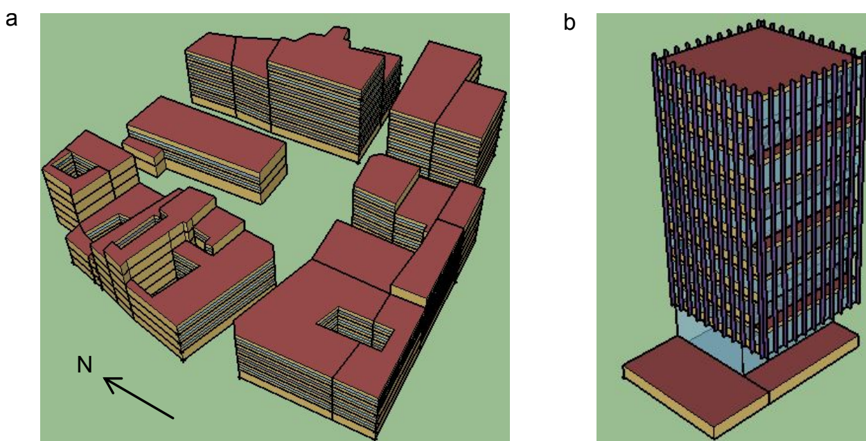
Figure III.4 - Modèles ED (a) et P (b) réalisés avec le plug-in d'OpenStudio pour SketchUp.
