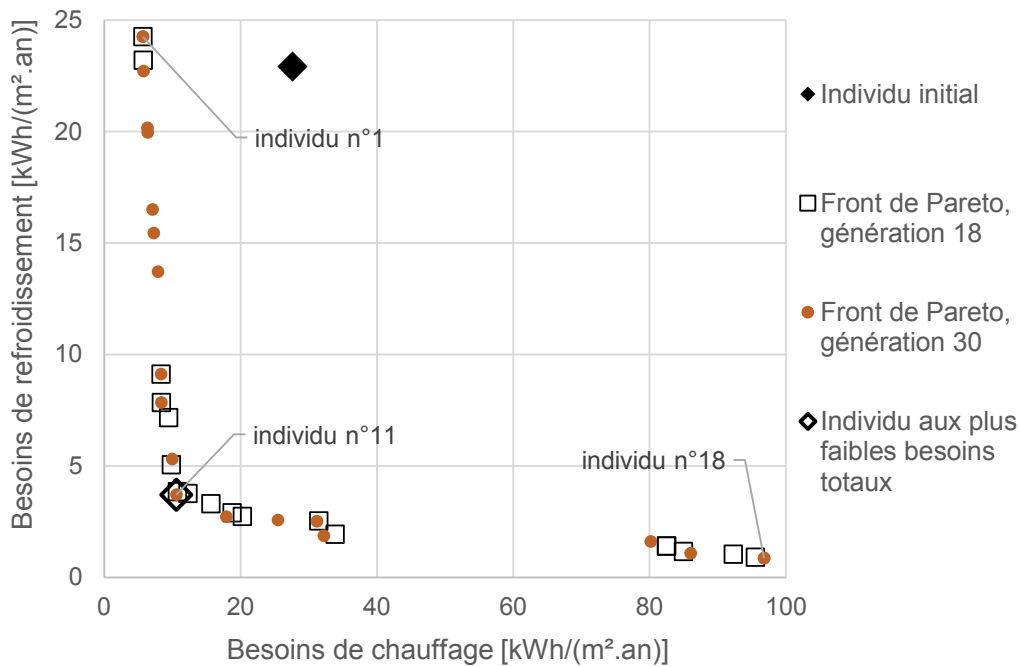
Figure IV.19 – Optimisation n°4 : individu initial, avant optimisation et fronts de Pareto obtenus pour la population des générations 18 et 30.
