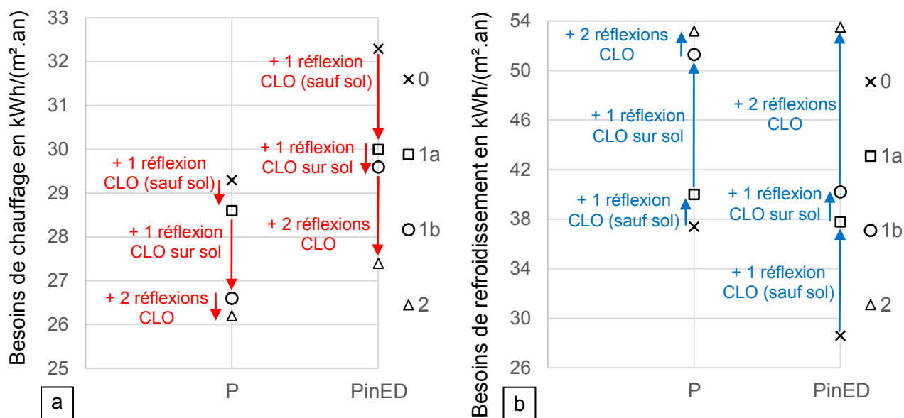
Figure III.15 – Comparaisons des besoins de chauffage (a) et de refroidissement (b) du bâtiment neuf obtenus avec la PFM pour les différentes versions des modèles P et PinED.
