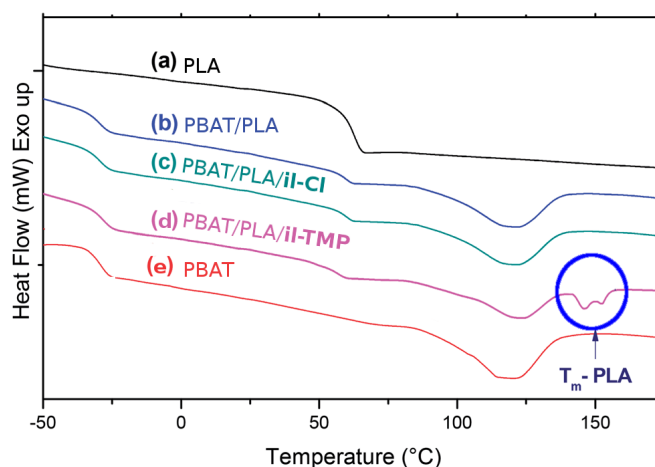
Figure 5 – Thermogrammes DSC de (a) PLA, (b) PBAT/PLA, (c) PBAT/PLA/IL-Cl, (d) PBAT/PLA/IL-TMP et (e) PBAT (Rampe: 10^\circ\text{C}\cdot\text{min}^{-1} ). Un phénomène de fusion, entouré en bleu, traduit l'apparition d'une phase cristalline dans le mélange PBAT/PLA/il-TMP, et la température d'environ 150^\circ\text{C} le fait correspondre à la phase PLA.
