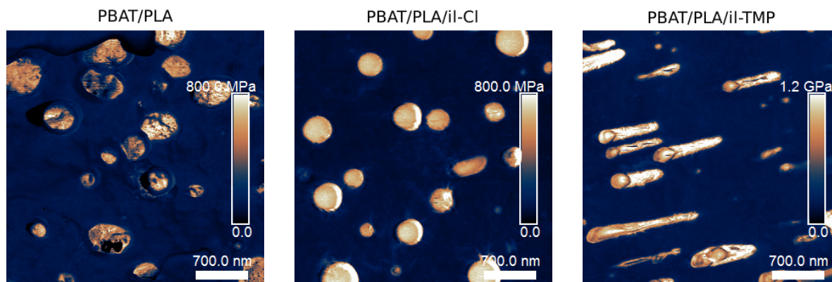
Figure 4 – Images AFM en module DMT ( 3.5 \times 3.5 \mu\text{m} ) de la microstructure du PBAT/PLA (gauche), du PBAT/PLA/il-Cl (centre) et du PBAT/PLA/il-TMP (droite).
