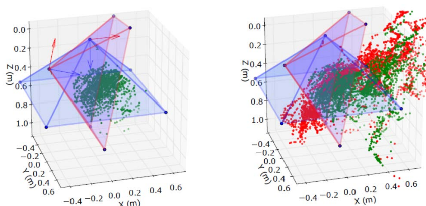
Figure A.6 – Gain en volume de travail de MonSterTrack et CoCaTrack (droite) par rapport à un système stéréo standard (gauche): Les points rouges représentent les objets localisés en monoculaire et les points vert en stéréo. La caméra bleue est contrôlée grâce à un moteur pan-tilt. La caméra rouge est fixe.
