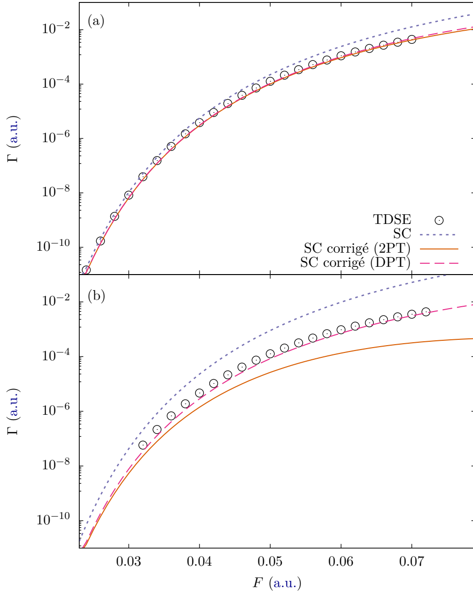
Figure S.3 Rendement d'ionisation tunnel de systèmes modèles à une dimension représentant des molécules diatomiques homonucléaires alignées avec le champ définis par un potentiel Soft-Coulomb(II.2) avec les paramètres (a) a = 1 u.a. et R = 2.2 u.a. (b) a = 0.6925 u.a. et R = 4 u.a..
