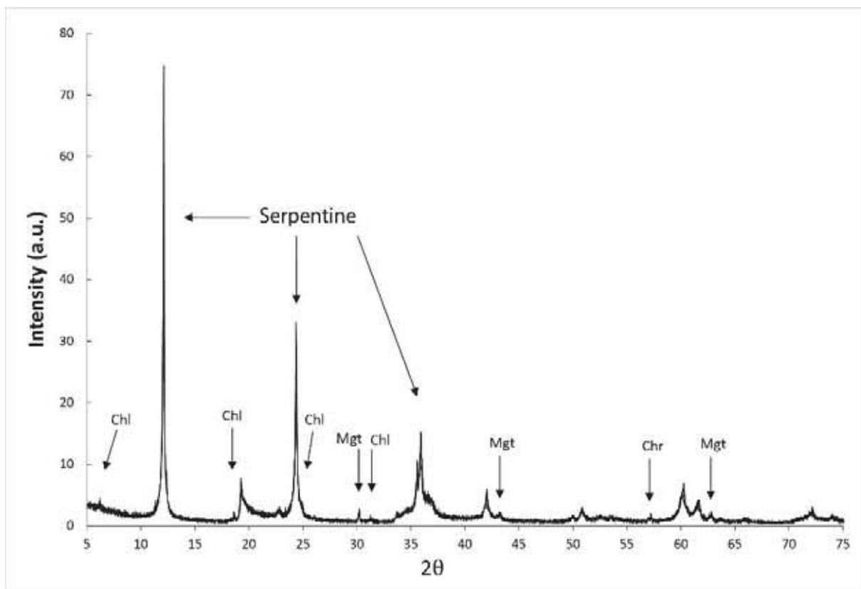
Figure I-39 : Exemple de diffractogramme pour une analyse de diffraction des rayons X réalisée sur une serpentinite de l'unité ultramafique d'Ait Ahmane (Ophiolite de Bou Azzer, Anti-Atlas, Maroc), permettant l'identification de lizardite et de chrysotile comme phases de serpentine et de chlorite (Chl), magnétite (Mgt) et chromite (Chr) comme phases accessoires (Hodel et al., 2017). Les piques de référence pour chaque espèce minérale sont disponibles sur la base de données RRUFF.info .
