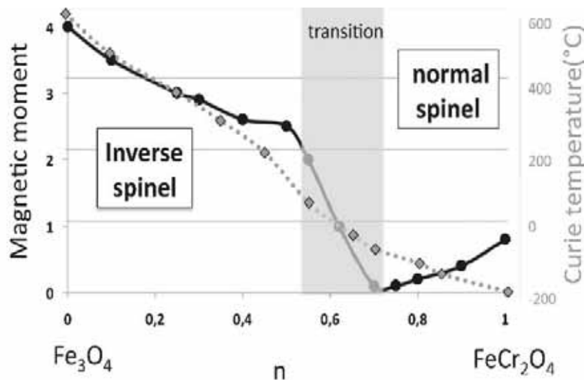
Figure IV-2 : Moment magnétique et températures de curie (décrites par la suite) pour la série des spinelles de type \text{Fe}^{2+}(\text{Fe}_{1-n}\text{Cr}_n)_2\text{O}_4 entre le pôle chromite ( \text{FeCr}_2\text{O}_4 , n=1 ) et le pôle magnétite ( \text{Fe}_3\text{O}_4 , n=0 ). Ferritchromite et magnétite chromifère sont des intermédiaires entre ces deux pôles purs. Par Horen et al. (2014), d'après Dunlop & Ozdemir, (1997) ; Ziemniak & Castelli, (2003) ; Kadzialko-Hofmohl et al. (2008).
