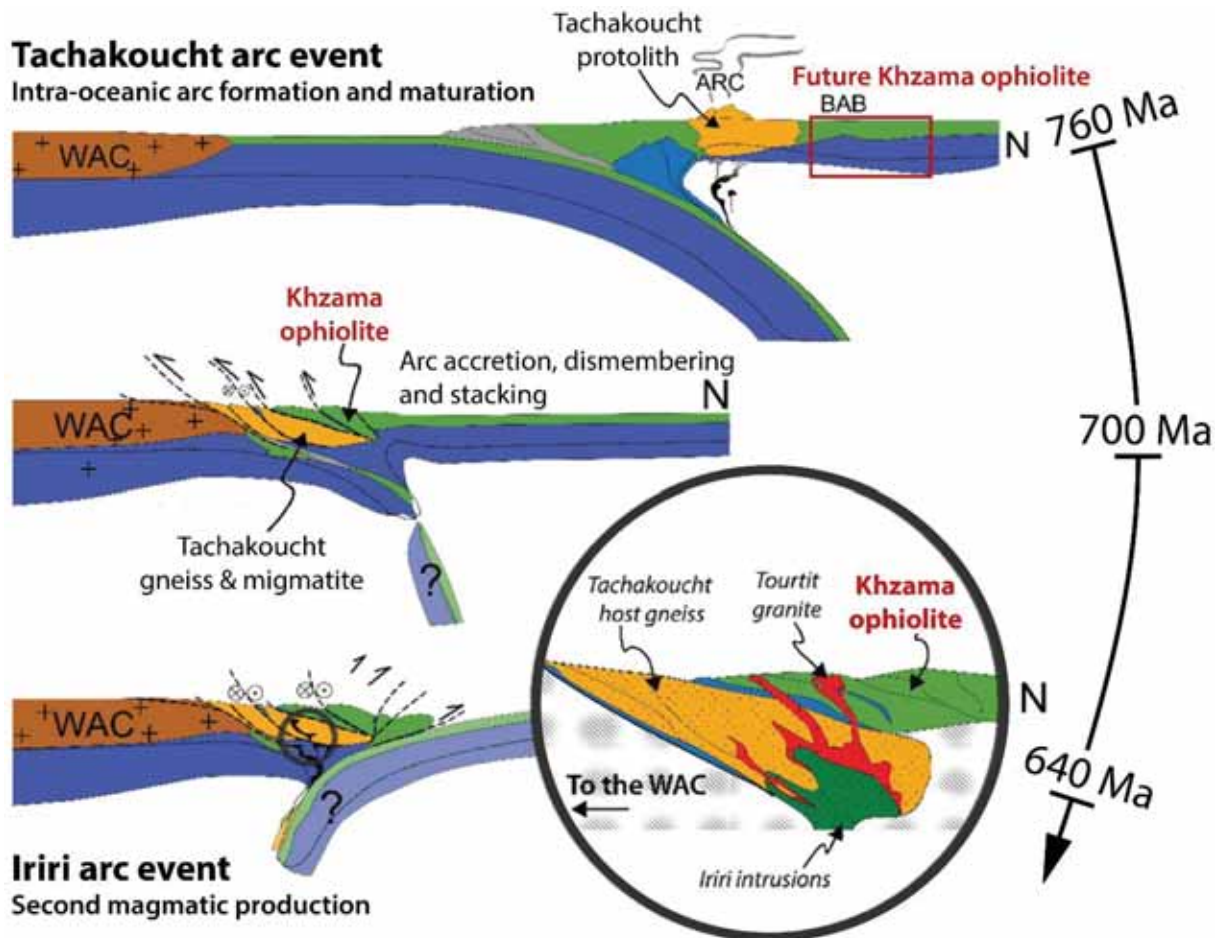
Figure II-4 : Modèle schématique de l'évolution du complexe d'arc océanique d'Iriri-Tachakoucht-Tourtit, modifié d'après Triantafyllou (2016). BAB : bassin arrière arc, back arc basin ; WAC : craton Ouest Africain, West African Craton .
