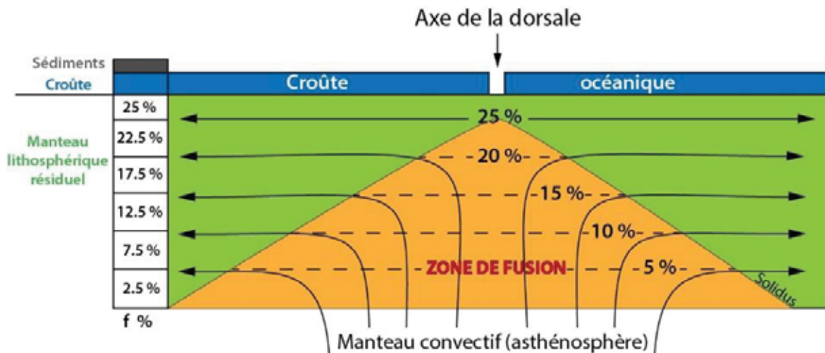
Figure I-20 : Représentation schématique de la fusion et de la stratification du manteau à l'aplomb d'une dorsale médio-océanique. Les péridotites sont de plus en plus réfractaires vers le haut de la colonne mantellique où les taux de fusion sont plus importants. D'après Plank & Langmuir (1992).
