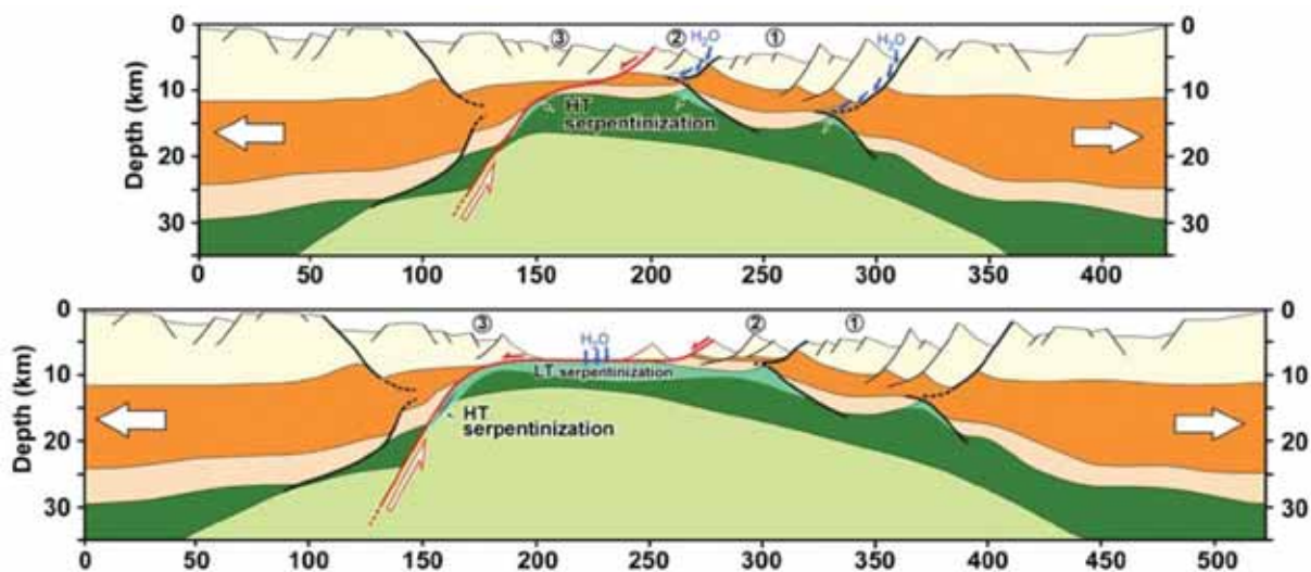
Figure I-46 : Schéma conceptuel de la formation d'une marge hyper-étendue, ainsi que de la mise à l'affleurement et de la serpentinisation des roches mantelliques associées. Par Guillot et al. (2015).
