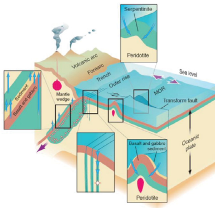
Figure I-43 : Représentation schématique des principaux contextes propices à la serpentinisation (Kerrick, 2002). De droite à gauche : Serpentinisation à l'axe des dorsales médio-océaniques, au niveau de failles transformantes. / Serpentinisation au niveau de champs hydrothermaux à l'axe des dorsales. / Serpentinisation via des failles normales associées à la flexure de la plaque plongeante au niveau des fosses de subduction. / Serpentinisation du coin mantellique par les fluides issus de la déshydratation de la plaque subduite en contexte de subduction.
