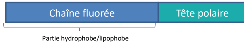
Figure II-3 : Schéma des perfluorocarbones
