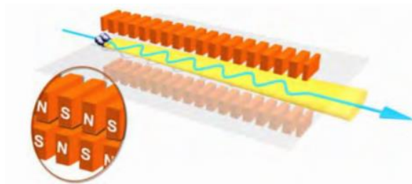
Figure IV-9 : Schéma d'un élément magnétique d'insertion
