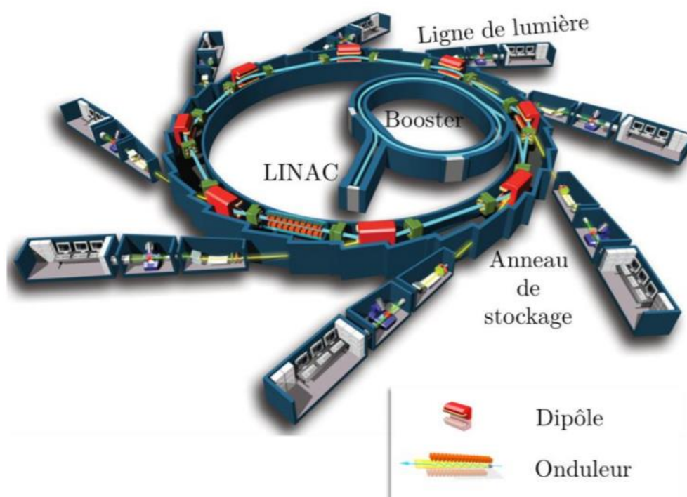
Figure IV-8 : Schéma du synchrotron SOLEIL et de la circulation des électrons à partir du canon à électrons jusqu'aux lignes de lumière
