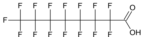
Figure II-5 : Structure développée de l'acide perfluorooctanoïque (PFOA) C_8HF_{15}O_2
