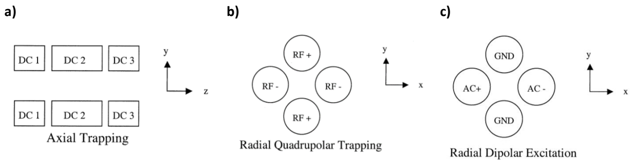
Figure IV-23 : Schéma d'application des tensions a) continues, b) de piégeage RF et c) alternative, nécessaire au fonctionnement du piège à ions 2D. Source : Schwartz et al. 137
