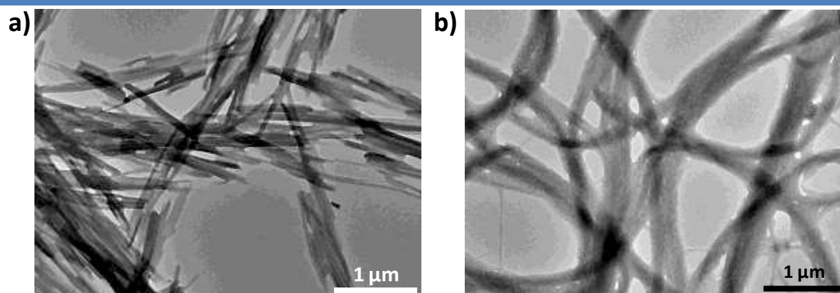
Figure 4. Images TEM de l'auto-assemblage des molécules a) TAMT en présence de mélamine dans le toluène et b) TAMG en présence de KPF_6 dans le toluène.
