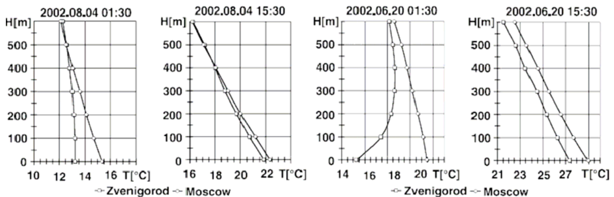
Figure 1.6 : Allure de la variation de la température en fonction de la hauteur à Moscou (zone urbaine) et Zvenigorod (zone environnante) pour 4 aout 2002 et 20 juin 2002 (Khaikine, et al., 2006).
