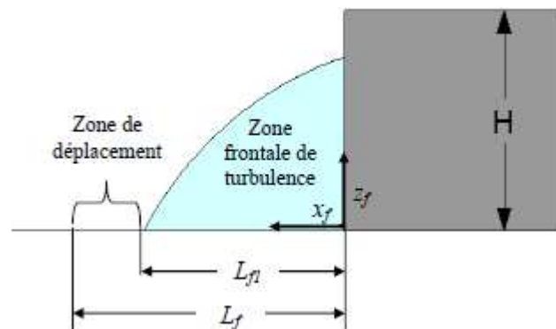
Figure 1.24 : Les différentes paramètres de la cavité frontale (Gros, 2013)
