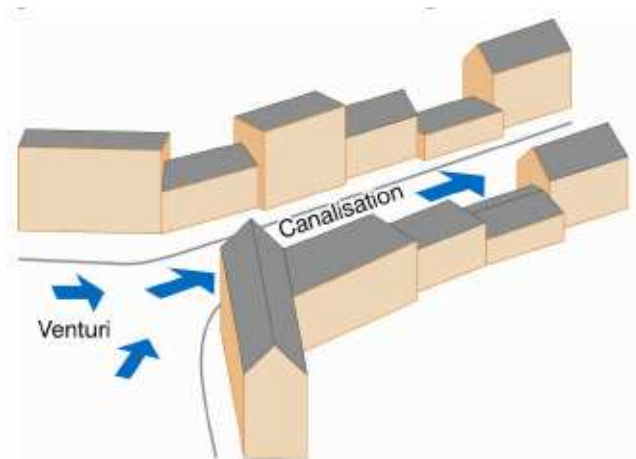
Figure 1.26 : Quelques effets aérodynamiques observés dans la configuration urbaine (Gandemer, 1975)
