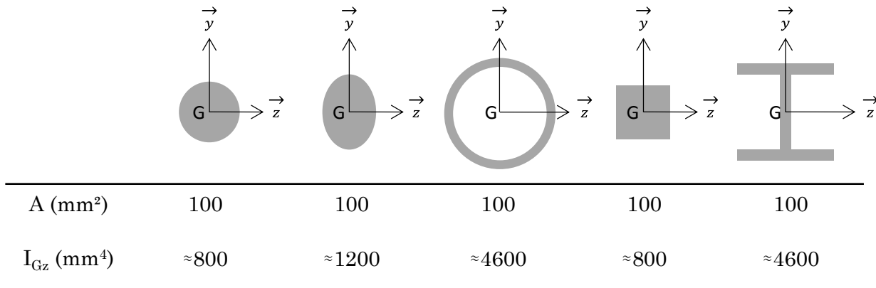
Figure 9. Moment quadratique selon l'axe Gz ( I_{Gz} ) pour des sections d'aire similaires ( A ) et de géométries différentes : tube plein de section circulaire, tube plein de section elliptique, tube creux, poutre pleine et poutre en I.
