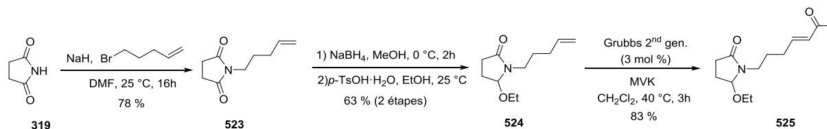
Schéma 150 : synthèse de l'ANF 525
