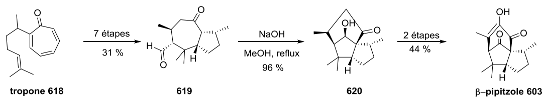
Schéma 190 : synthèse du β-pipitzole par une réaction d'aldolisation intramoléculaire
