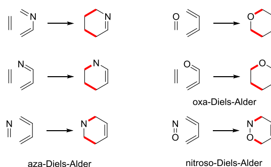
Figure 7 : réaction d'hétéro-Diels-Alder
