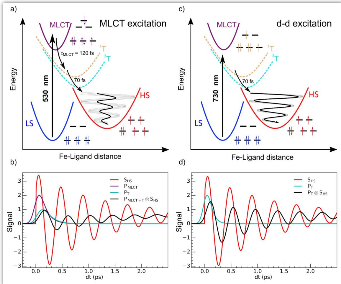
Figure 2 : Comparaison des processus LIESST avec l'excitation MLCT et d-d
