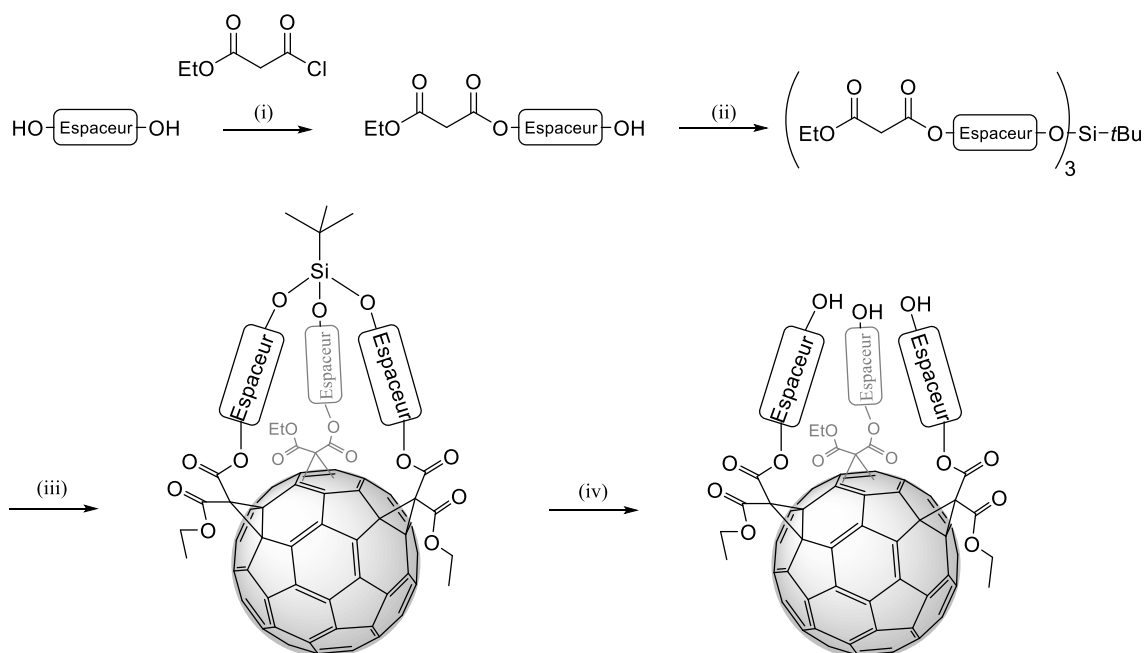
Figure 6 : Réactifs et conditions : (i) pyridine, THF, 0^\circ\text{C} à t.a., 12 h; (ii) t\text{BuSiCl}_3 , imidazole, DMF, t.a., 12 h; (iii) C_{60} , I_2 , DBU, toluène, -15^\circ\text{C} , 1 h.
