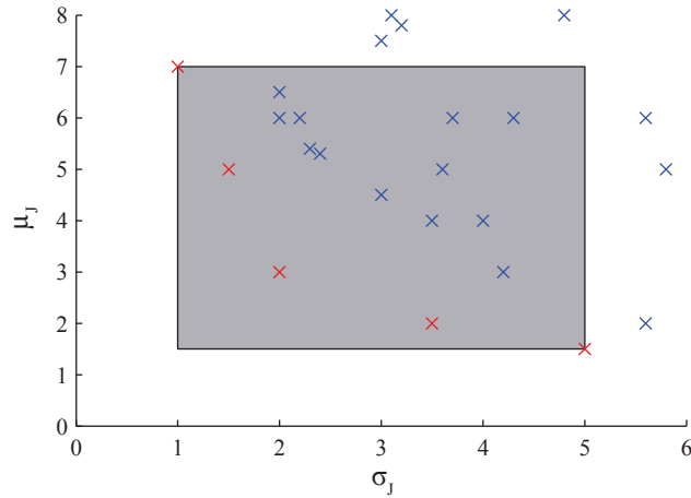
FIGURE 3.12 – Zone d'analyse autour du front de Pareto fréquentiel
