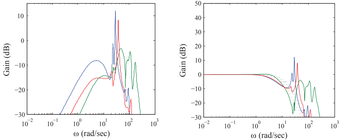
(a) Erreur entre modèle de référence et le système M_0 - T et pondération W_p
