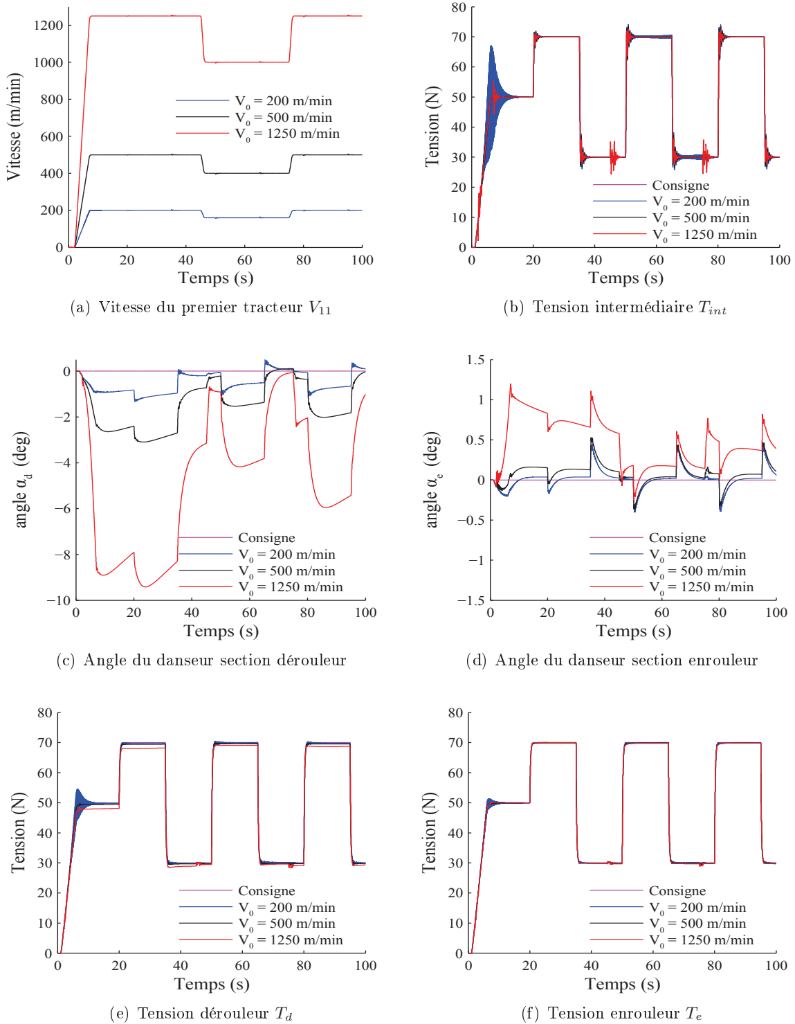
FIGURE 2.17 – Simulation du modèle non-linéaire pour plusieurs valeurs de la vitesse de défilement
