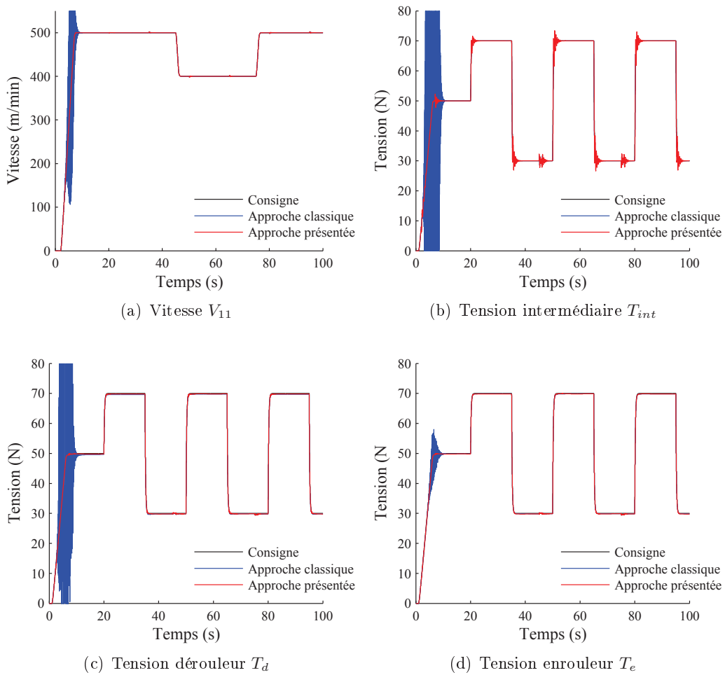
FIGURE 3.10 – Comparaison entre les approches fréquentielle et classique pour Ex2
