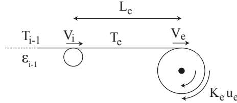
FIGURE 1.5 – Schéma de l'enrouleur axial
