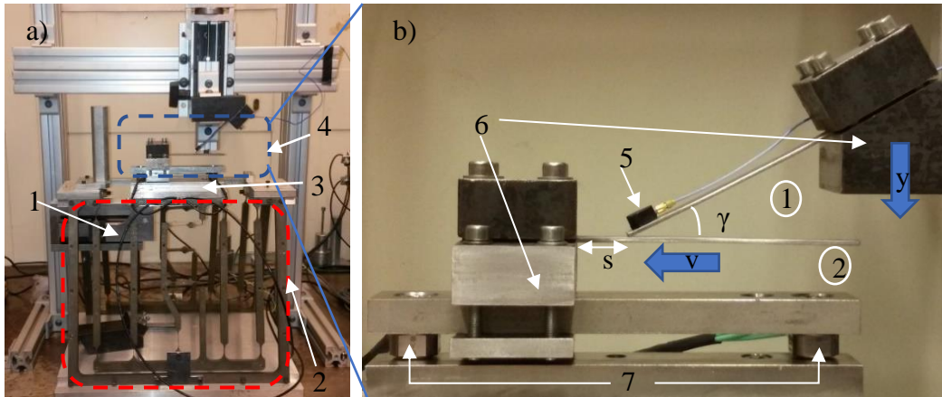
Figura 1: a) set.up TriboTouch, (1) coppia bobina-magnete, (2) dispositivo compliant, (3)base superiore,(4) sistema di bloccaggio delle travi; b) ingrandimento del set-up sul sistema di bloccaggio delle travi, (5) accelerometro, (6) masse di bloccaggio, (7) trasduttori di forza.
