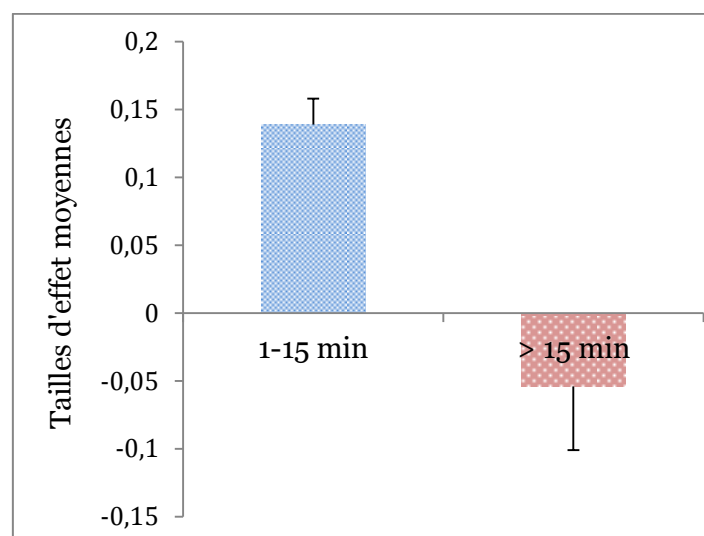
FIGURE 2 – Tailles d'effet de l'exercice sur la performance cognitive en fonction du délai entre la fin de l'exercice et la passation de la tâche cognitive (1-15 minutes vs supérieur à 15 minutes). Les barres d'erreurs représentent les erreurs standards. (Données issues de Chang et al. 2012).
