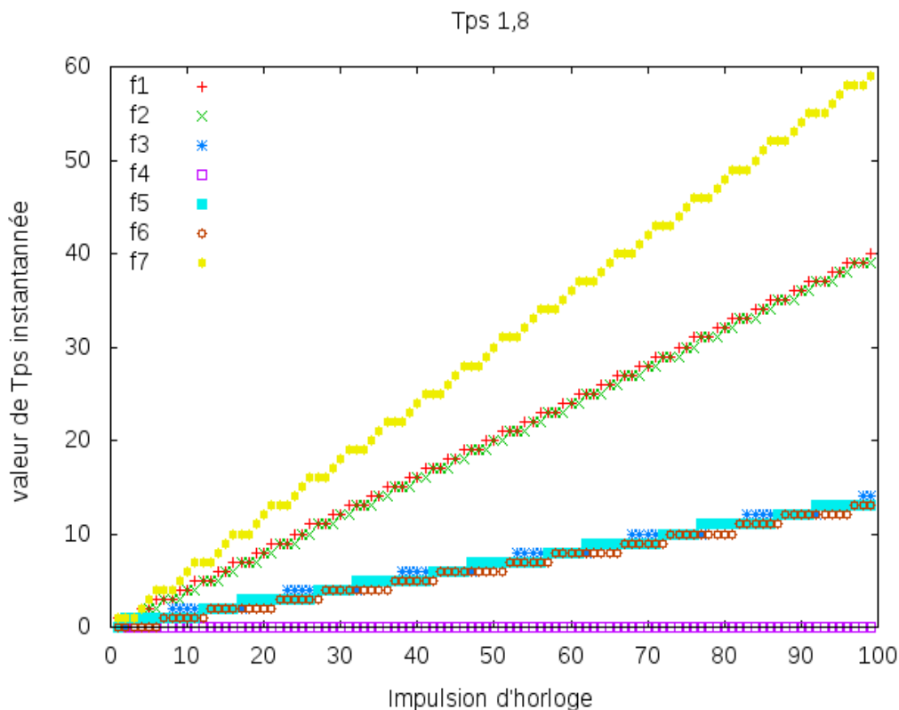
FIGURE 3.7 – Nombre de paquets émis pour TpsW = 1.8
