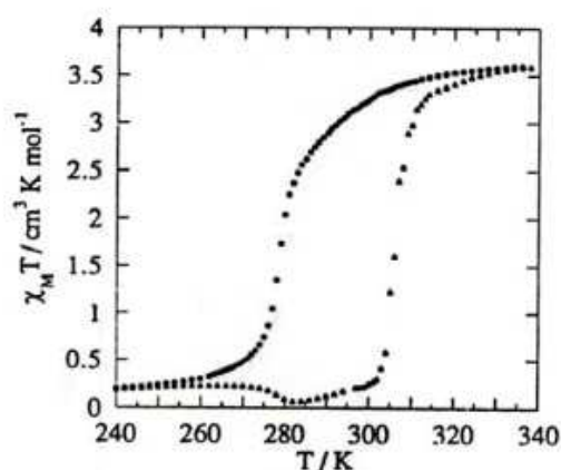
Figure 1.5. Produit \chi_m T en fonction de la température pour le complexe [\text{Fe}(\text{NH}_2\text{trz})_3](\text{Br})_2 \cdot \text{H}_2\text{O} . 28
