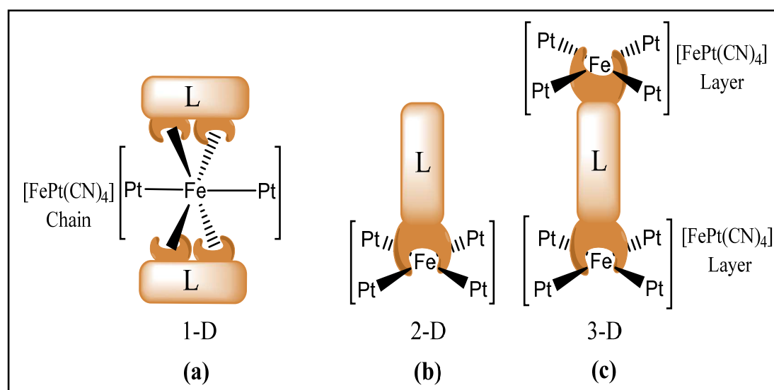
Schéma V.1. Exemple de stratégie utilisée pour la conception des systèmes à dimensions variées.
