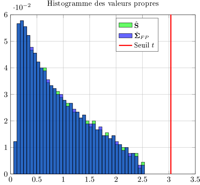
FIGURE 2.8 – Distribution des valeurs propres des matrices \hat{\mathbf{S}} et \check{\Sigma}_{FP} ainsi que le seuil t pour \rho = 0.7 , m = 900 , N = 2000 , \tau \sim inverse gamma.
