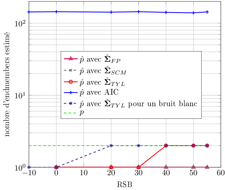
FIGURE 3.9 – Estimation du nombre d' endmembers \hat{p} pour un bruit CES corrélé, m = 240 , c = 0.24 , p = 2 , \rho = 0.7 , \{\tau\} \sim inverse gamma , en fonction du RSB.
