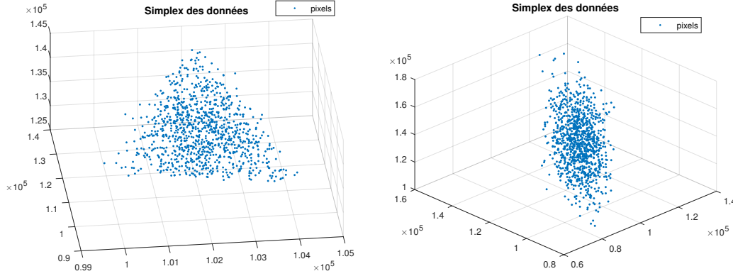
FIGURE 1.8 – Représentation des données dans un simplexe, N = 1000 , m = 900 , données corrélées.
