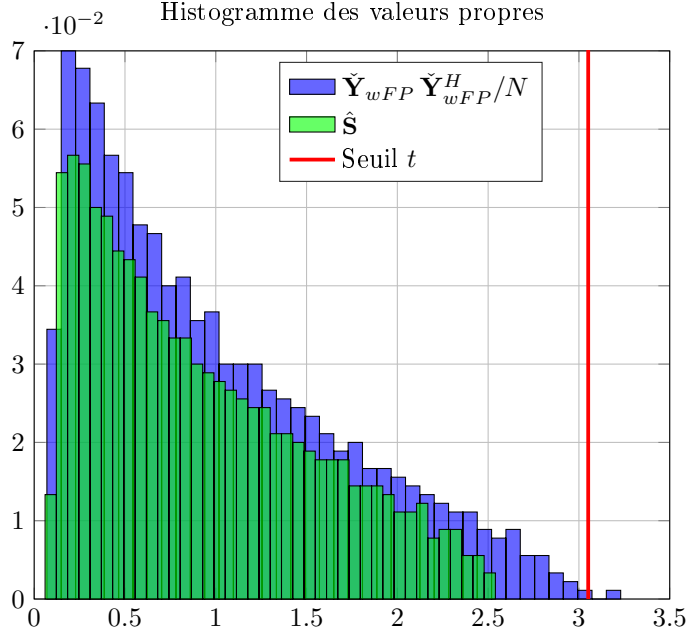
FIGURE 2.11 – Distribution des valeurs propres des matrices \hat{S} et de la matrice représentant la SCM de \check{Y}_{wFP} \check{Y}_{wFP}^H / N et le seuil t pour \rho = 0.7 , m = 900 , N = 2000 , \tau \sim inverse gamma.
