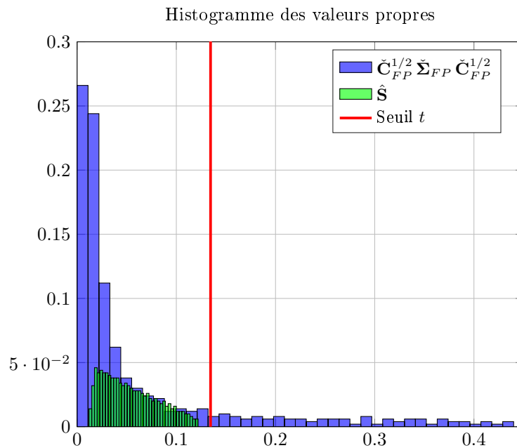
FIGURE 2.10 – Distribution des valeurs propres des matrices \hat{\mathbf{S}} et \tilde{\Sigma}_{FP} pour un signal non blanchi ainsi que le seuil t pour \rho = 0.7 , m = 900 , N = 2000 , \tau = t^2 , t \sim \text{Student} .
