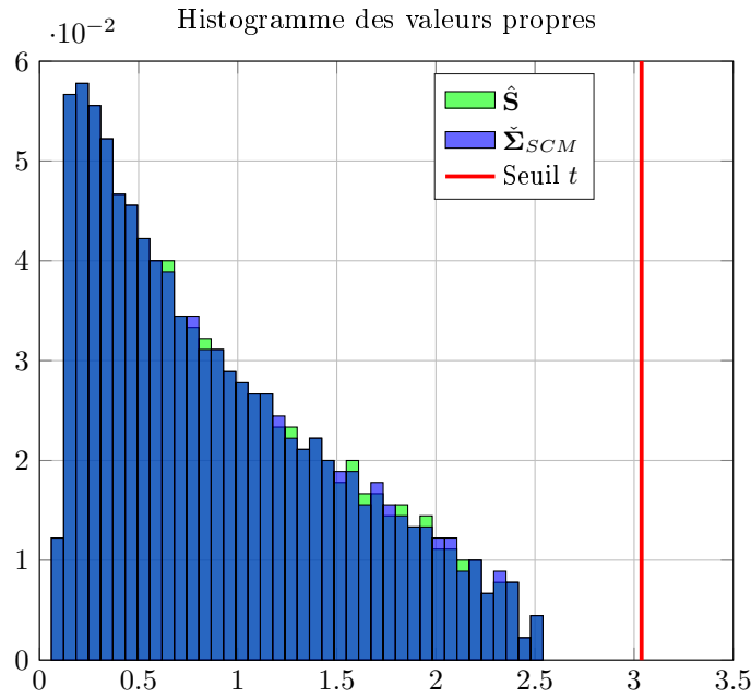
FIGURE 2.4 – Valeurs propres des matrices \tilde{\Sigma}_{SCM} et \hat{S} lorsque le signal \mathbf{Y} a été blanchi par \tilde{\mathbf{C}}_{SCM} et le seuil correspondant t pour \rho = 0.7 , m = 900 , N = 2000 , \tau = inverse gamma, \alpha = 0.1 , p = 0 .
