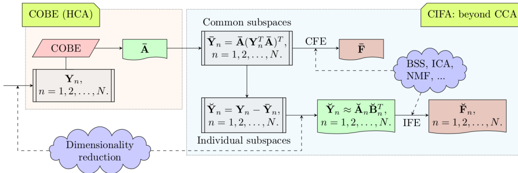
FIGURE 3.22 – Schéma d'extraction de CIFE (illustration provenant de [124]).
