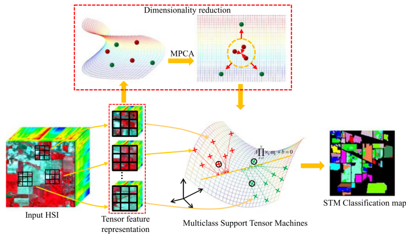
FIGURE 3.4 – Système de classification de données satellites par MPCA puis STM (illustration provenant de [36]).
