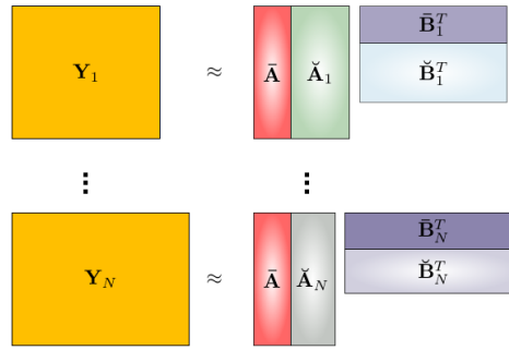
FIGURE 3.20 – Illustration de la formulation matricielle de CIFE (illustration provenant de [124]).
