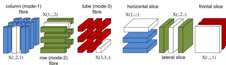
FIGURE 3.1 – Illustration des fibres et des tranches dans les tenseurs (illustration provenant de [48]).
