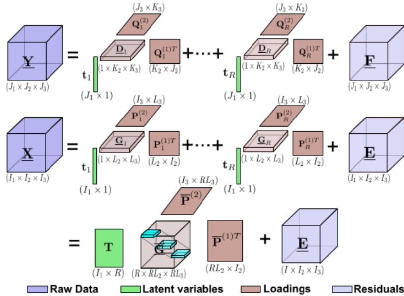
FIGURE 6.8 – Diagramme schématisé de la méthode HOPLS : l’approximation d’un tenseur \mathcal{X} par une somme de tenseurs de rang (1, L_2, L_3) et l’approximation de \mathcal{Y} suivant le même principe avec les composantes latentes communes T (illustration provenant de [121]).
