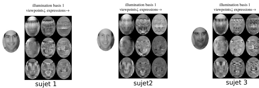
FIGURE 3.15 – Les premiers vecteurs propres selon le sujet 1, 2 et 3 en suivant les dimensions des points de vue et des expressions faciales (illustration de [102]).
