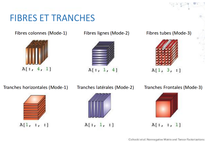
FIGURE 6.1 – Illustration des fibres et des tranches dans les tenseurs (illustration provenant de [15]).
