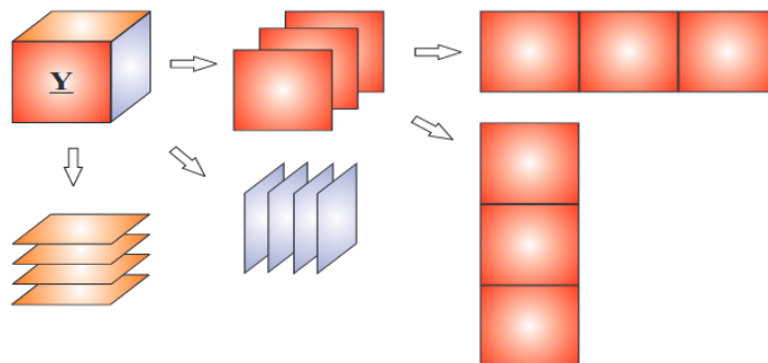
FIGURE 3.2 – Illustration des matricisations possibles d'un tenseur d'ordre 3 (illustration provenant de [15]).
