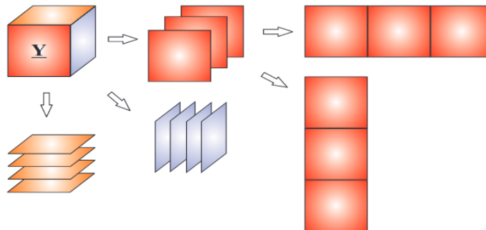
FIGURE 6.2 – Illustration des matricisations possibles d'un tenseur d'ordre 3 (illustration provenant de [15]).
