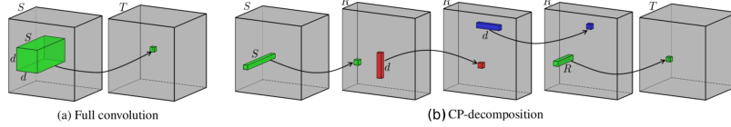
FIGURE 3.6 – Illustration d'une convolution classique dans un réseau de neurones (a) et la combinaison de 4 convolutions simples (illustration provenant de [59]).
