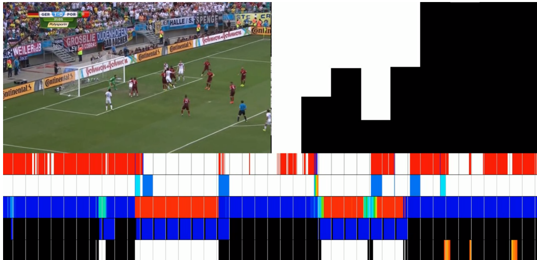
FIGURE 2.9 – En haut à gauche : image aléatoire d’un match de football. En haut à droite : son histogramme spatio-temporel. En bas : 5 frises qui décrivent les critères de détection de moments saillants (de haut en bas : zooms avant/arrière, le compteur de changement de zoom, la saturation, la détection de ralenti et le niveau d’activité).
