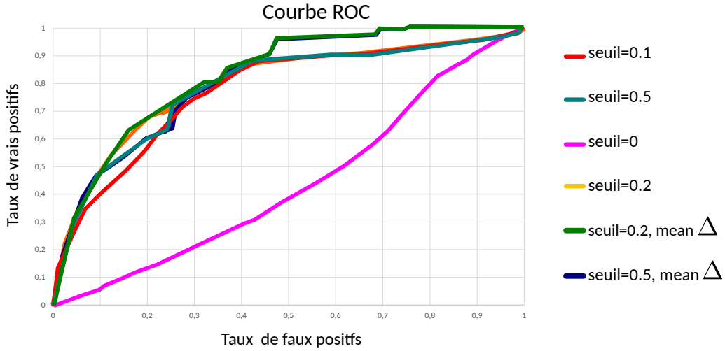
FIGURE 2.5 – Courbes ROC de notre méthode pour les différents seuils sur \det(\mathbf{A}) . Le meilleur résultat est obtenu avec un seuil de 0.2 sur \det(\mathbf{A}) et un \Delta(\mathbf{A}) moyenné sur 30 images.
