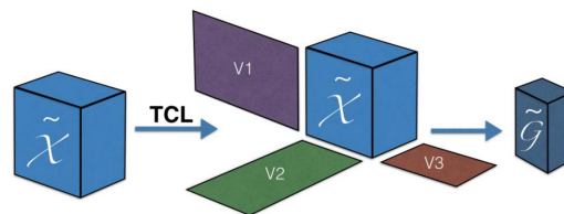
FIGURE 3.8 – Illustration d’une couche TCL sur un tenseur d’entrée d’ordre 3 (illustration provenant de [54]).
