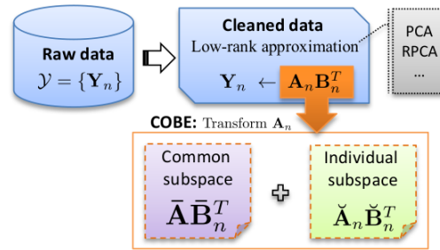
FIGURE 3.21 – Schéma d'extraction de CIFE (illustration provenant de [124]).
