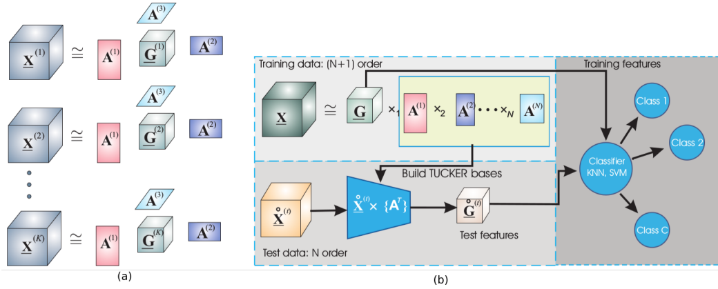
FIGURE 3.16 – (a) Illustration d'une extraction de représentation par TPCA. (b) Le système classique de classification par TPCA sur le tenseur contenant l'ensemble des données (illustration provenant de [78]).
