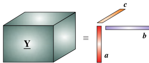
FIGURE 6.4 – Illustration d'un tenseur de rang 1 (illustration provenant de [15]).
