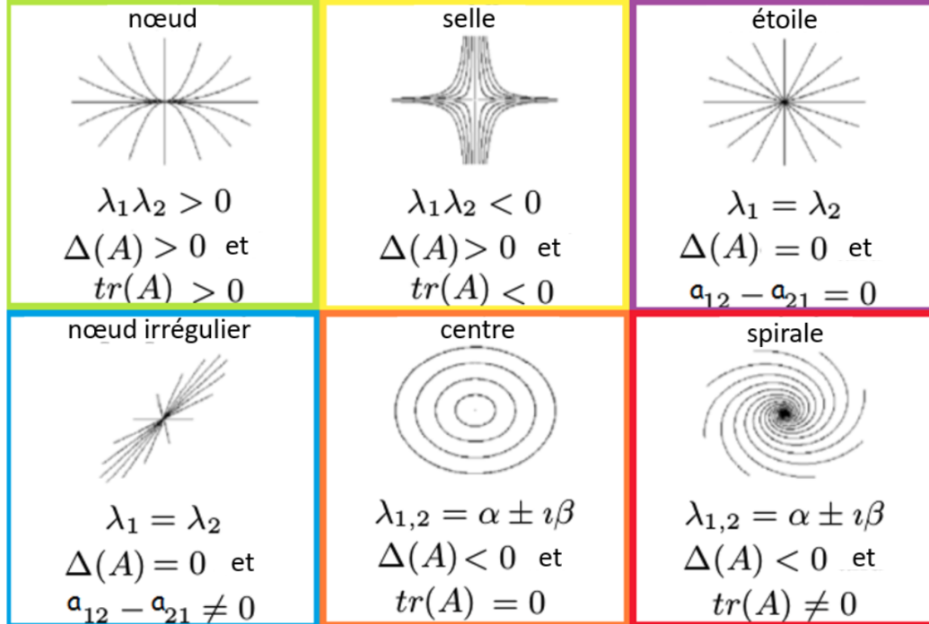
FIGURE 2.1 – Classification des singularités selon les valeurs de \mathbf{A} (illustration construite à partir d'une illustration provenant de [49]).
