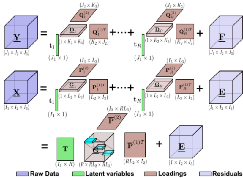
FIGURE 3.18 – Diagramme schématisique de la méthode HOPLS : l’approximation d’un tenseur \mathcal{X} par une somme de tenseurs de rang (1, L_2, L_3) et l’approximation de \mathcal{Y} suivant le même principe avec les composantes latentes communes T (illustration provenant de [121]).
