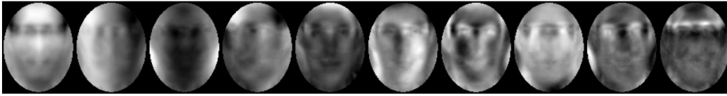
FIGURE 3.11 – Les 10 premières colonnes de U_{pixels} (illustration de [102]).
