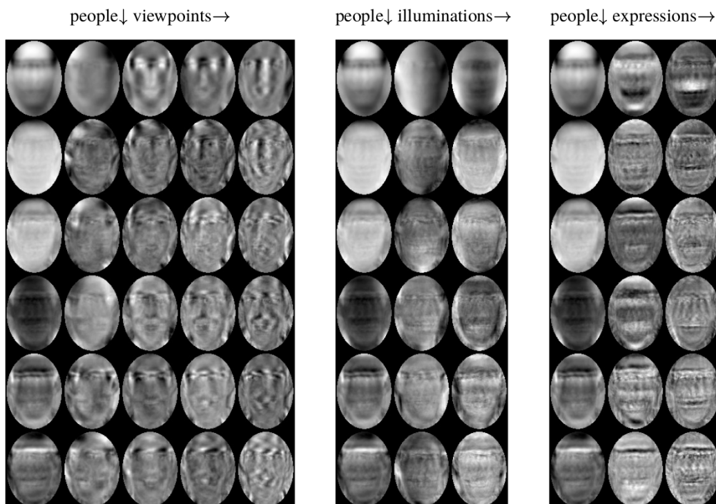
FIGURE 3.12 – Les premiers vecteurs propres contenus dans Z \times_5 U_{pixels} selon différentes directions (illustration de [102]).
