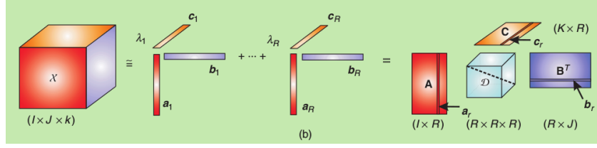
FIGURE 3.5 – Une décomposition CP d’un tenseur d’ordre 3 (illustration provenant de [14]).
