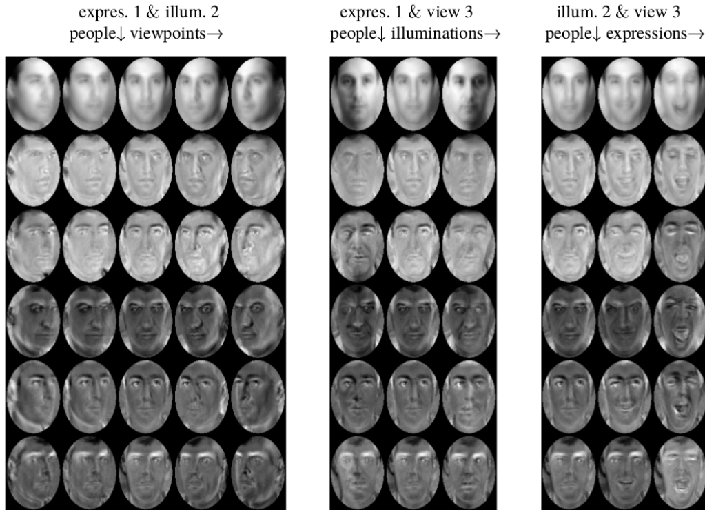
FIGURE 3.14 – Les premiers vecteurs propres en fixant tous les attributs sauf l’identifiant du sujet (illustration de [102]).
