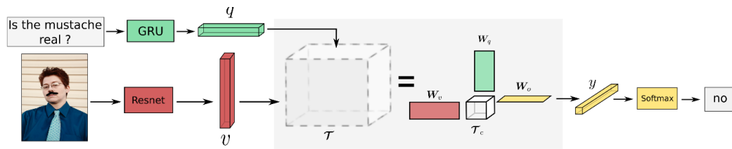
FIGURE 3.9 – Réseau de neurones MUTAN pour une application de réponse à une question à partir d’une image de [5]).
