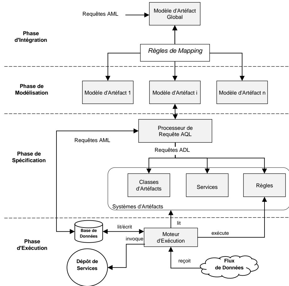
Figure 4. Cadre d'intégration de processus centré sur les artefacts
