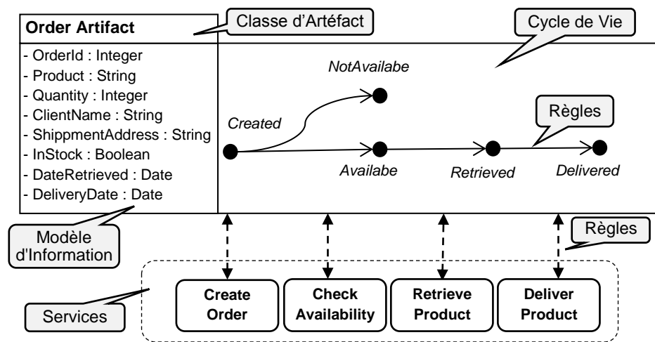
Figure 1. Exemple d'un Système d'Artéfacts
