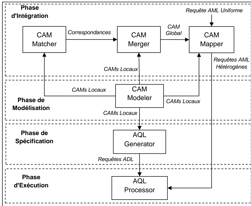
Figure 9. Modules principaux du prototype
