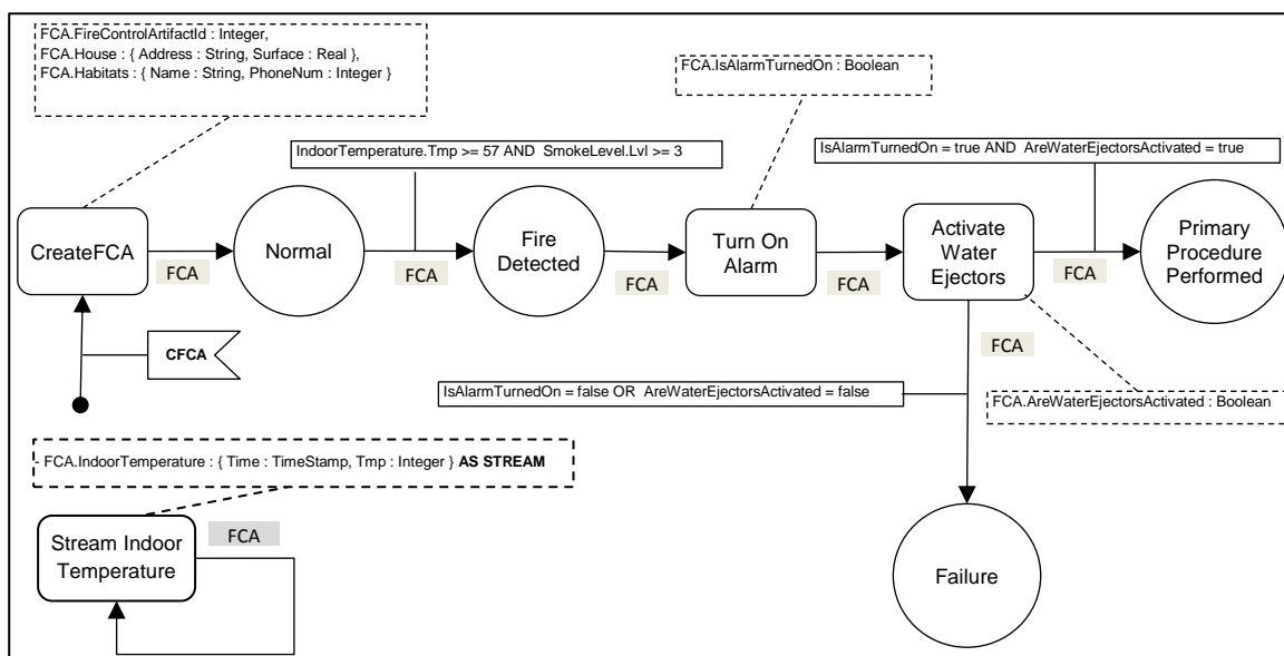
Figure 5. Partie du modèle d'artefact conceptuel d'un contrôle d'incendie
